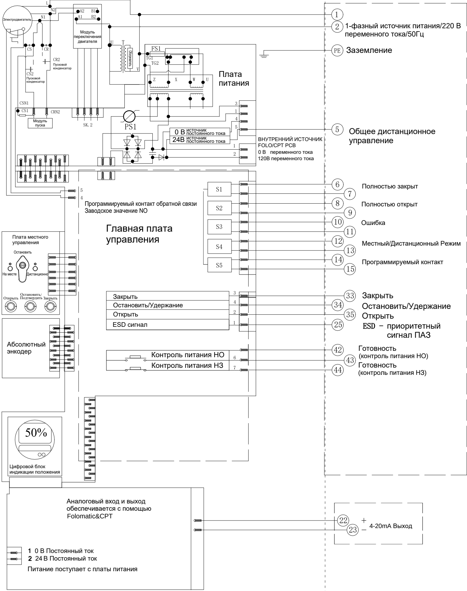
Электрическая схема №6-220-24-6-N-3 Серии VADM
