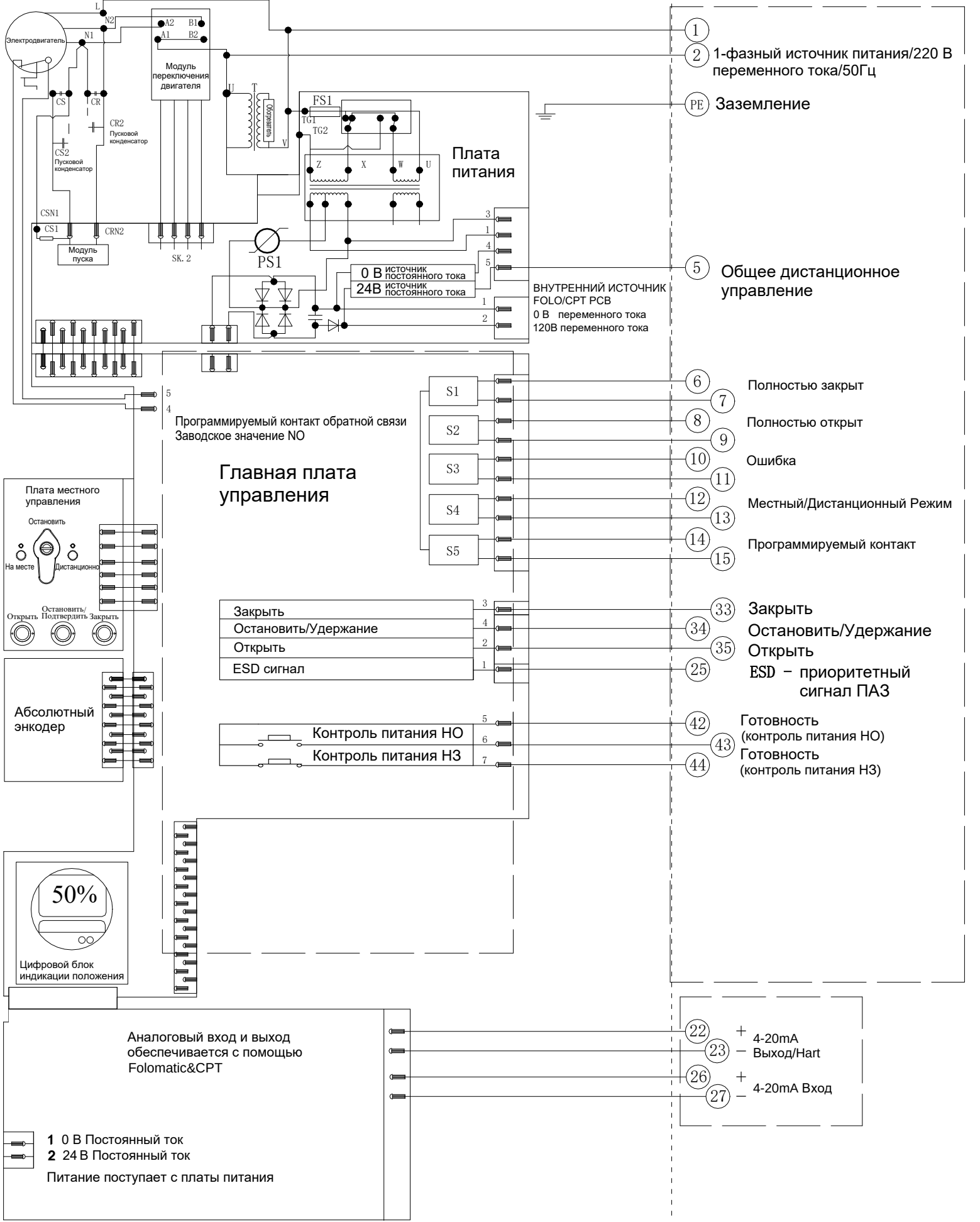
Электрическая схема №6-220-24-6-HR-1 Серия VADM
