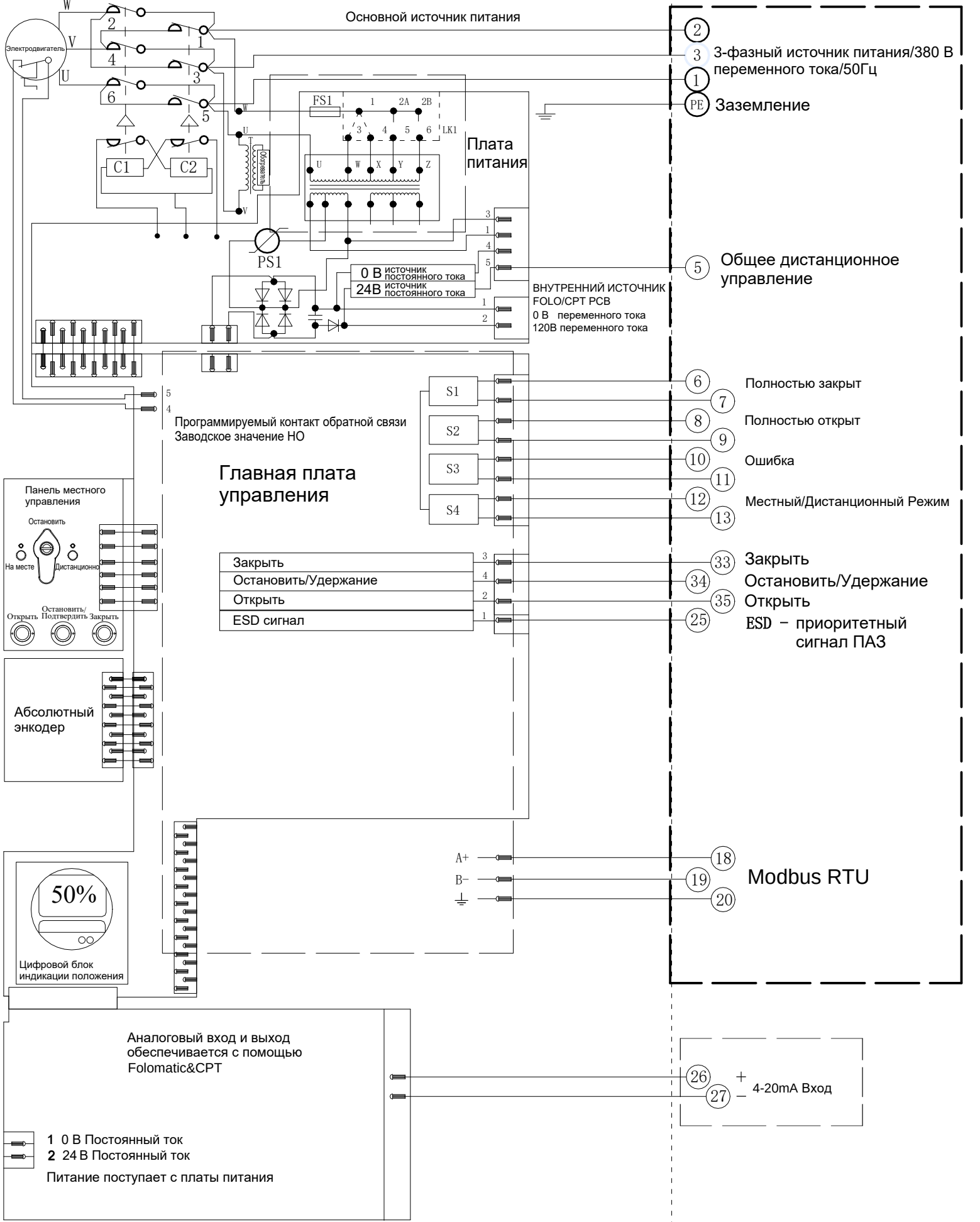
Электрическая схема №6-380-24-4-MR-2 Серия VADM
