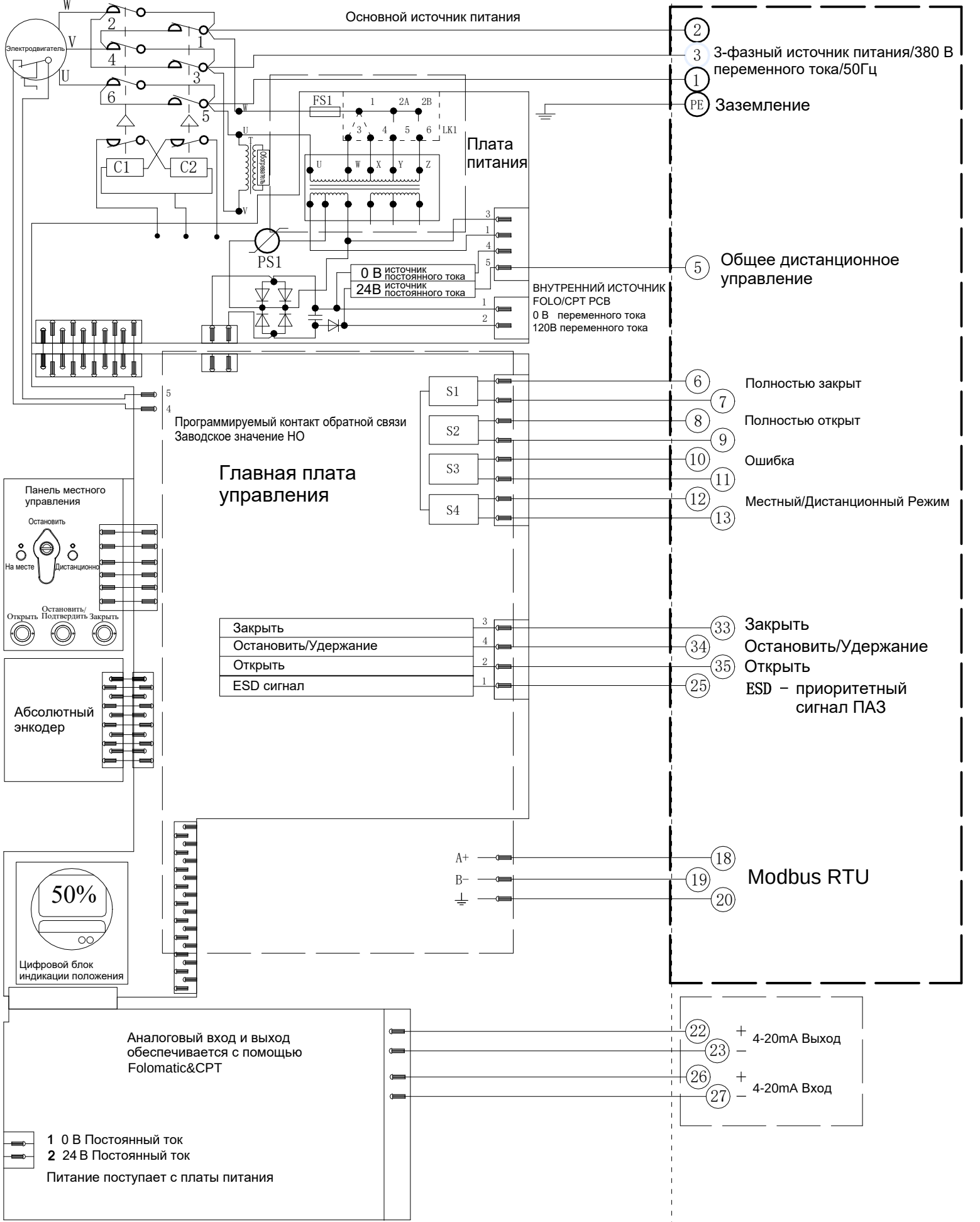
Электрическая схема №6-380-24-4-MR-1 Серия VADM
