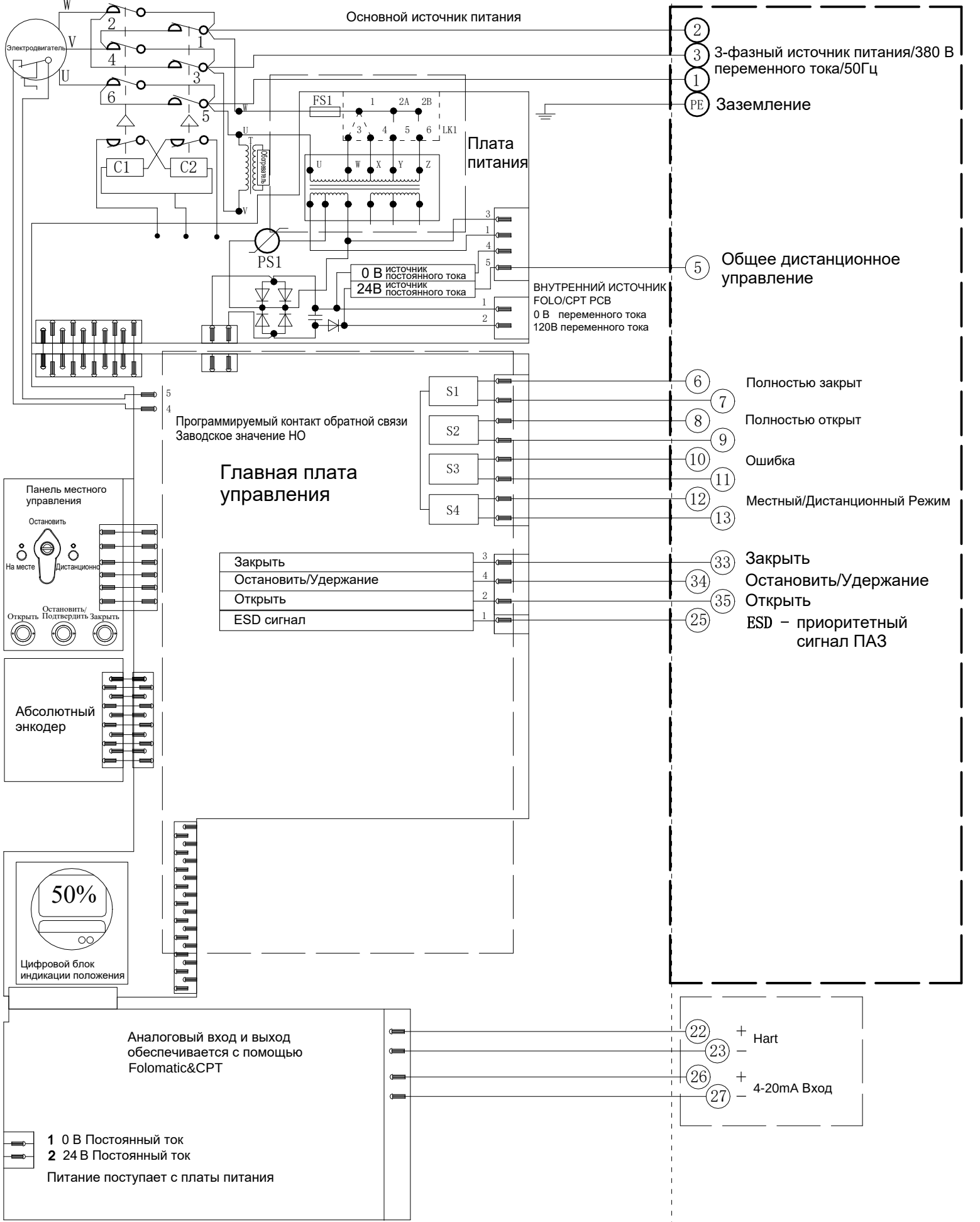
Электрическая схема №6-380-24-4-HR-2 Серия VADM
