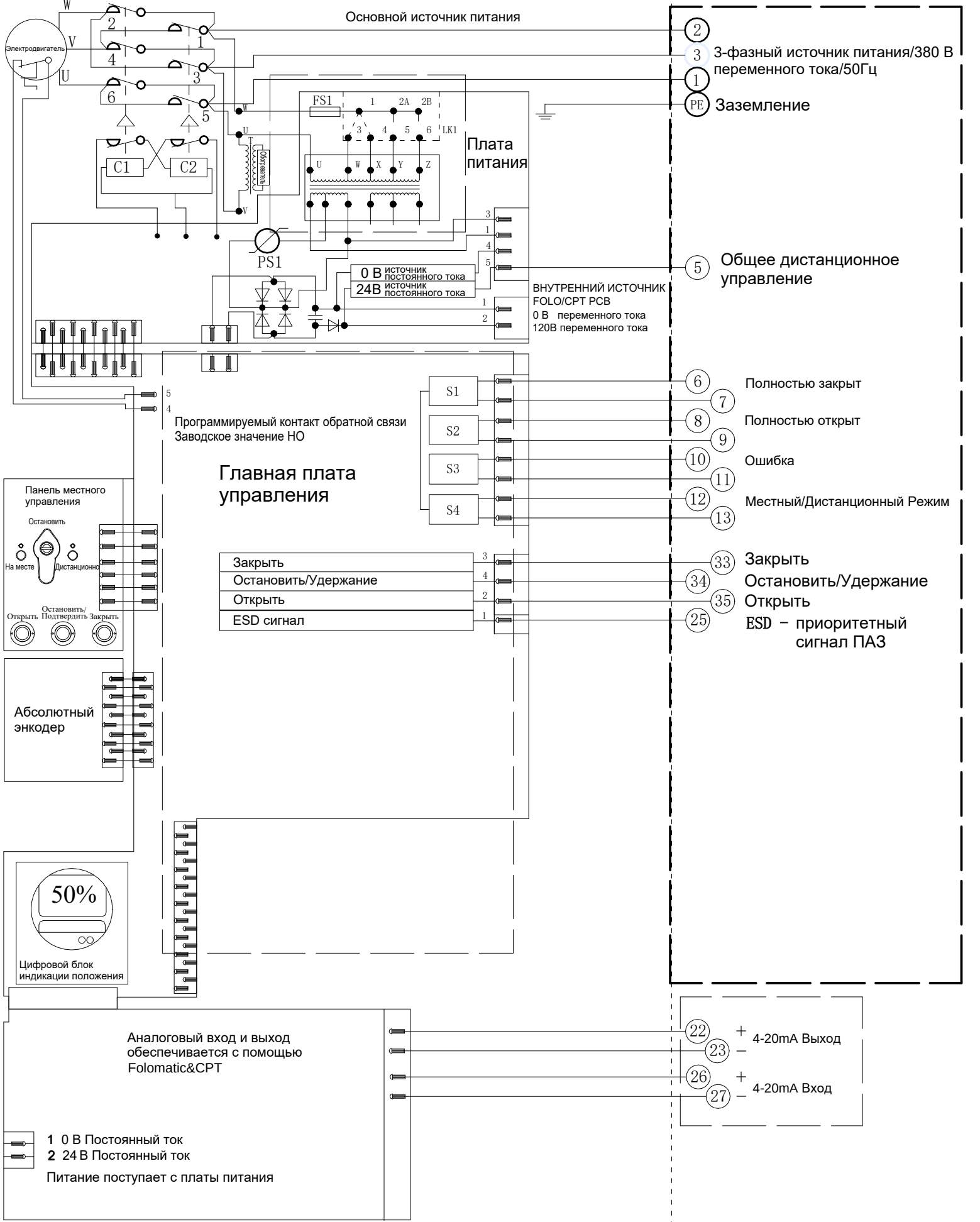
Электрическая схема №6-380-24-4-N-1 Серия VADM
