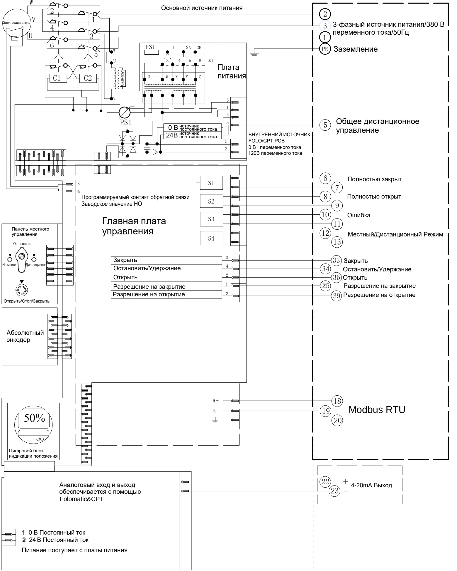
Электрическая схема №6-380-24-4-MR-3 Серия VADM
