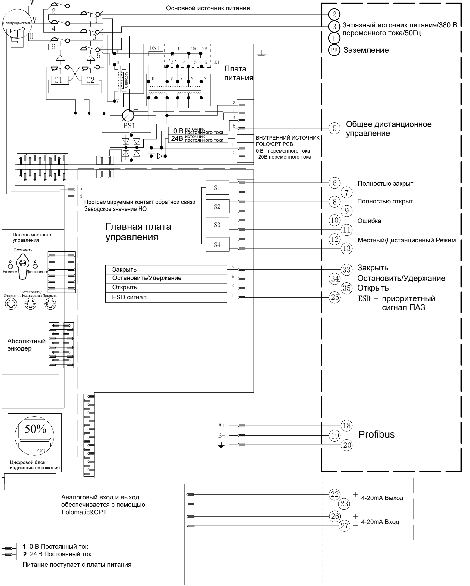
Электрическая схема №6-380-24-4-PR- 1 Серия VADM
