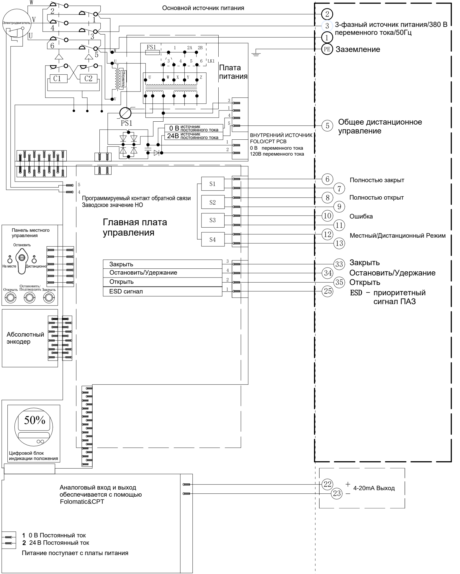
Электрическая схема №6-380-24-4-N-3 Серия VADM
