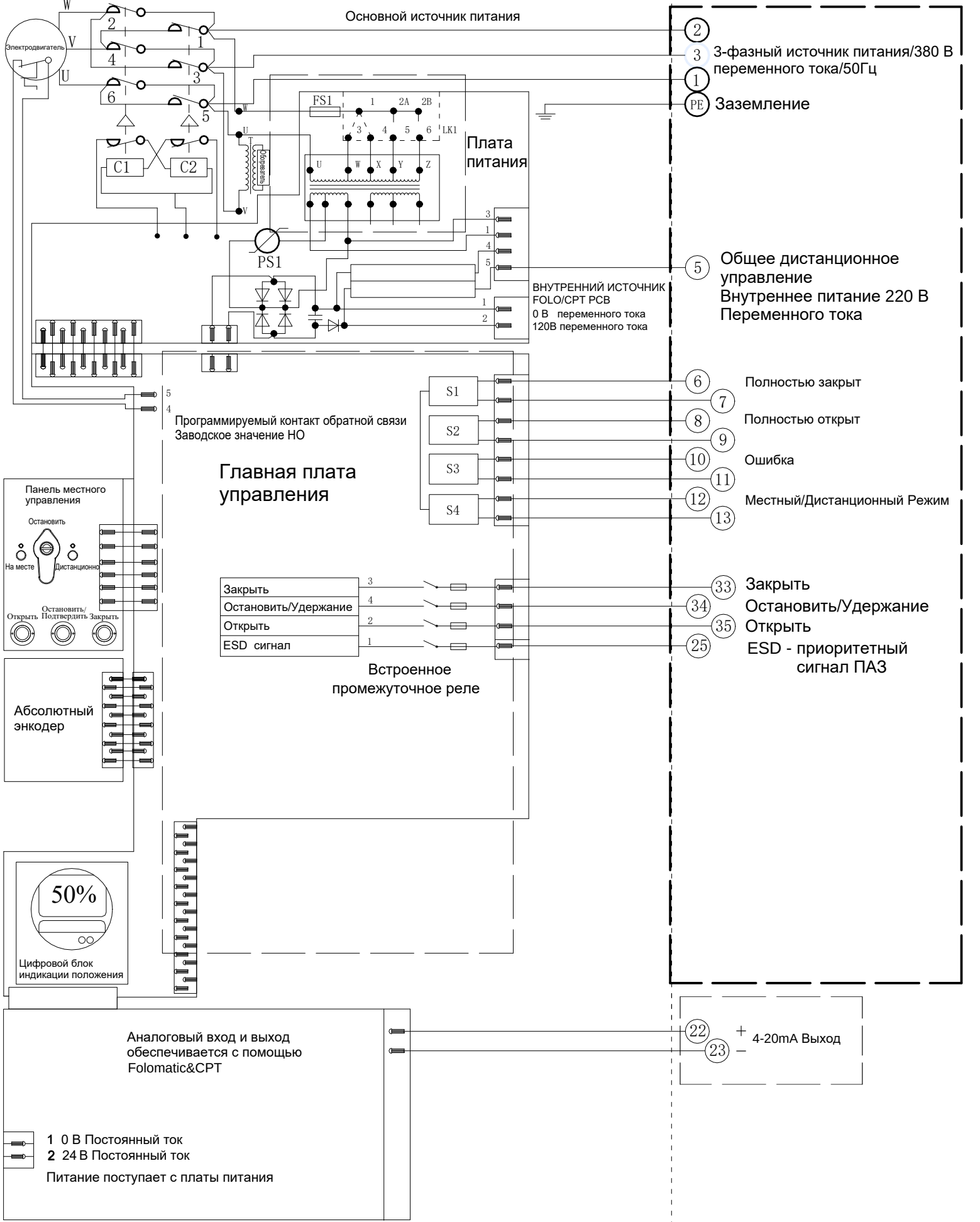
Электрическая схема №6-380-220-4-N-3 Серия VADM
