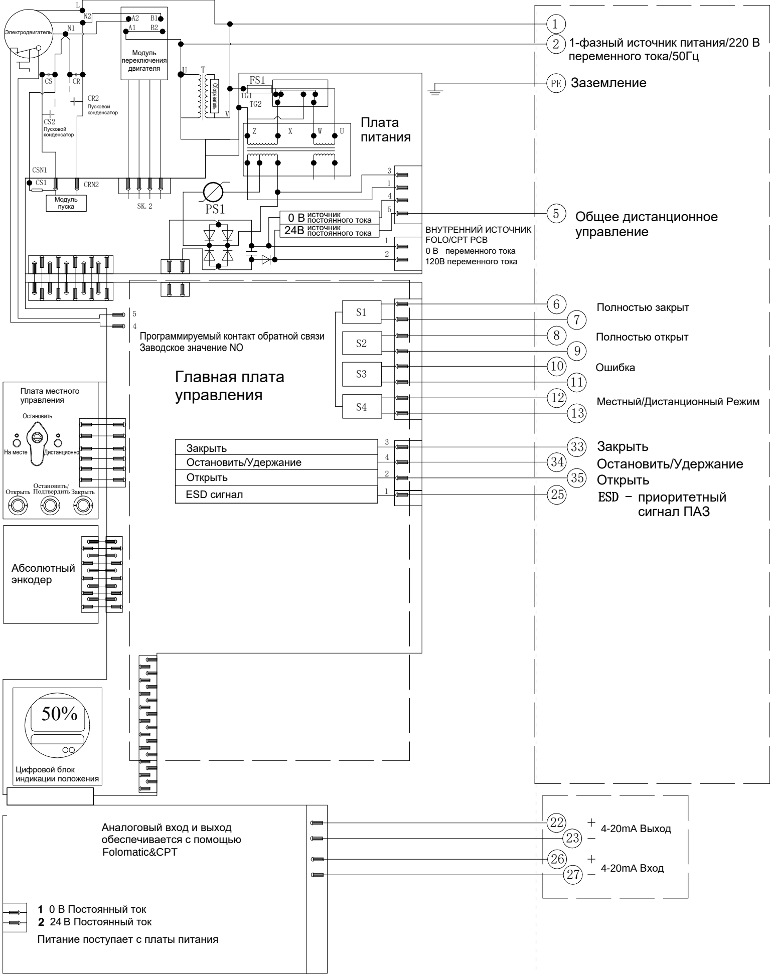
Электрическая схема №6-220-24-4-N-1 Серия VADM
