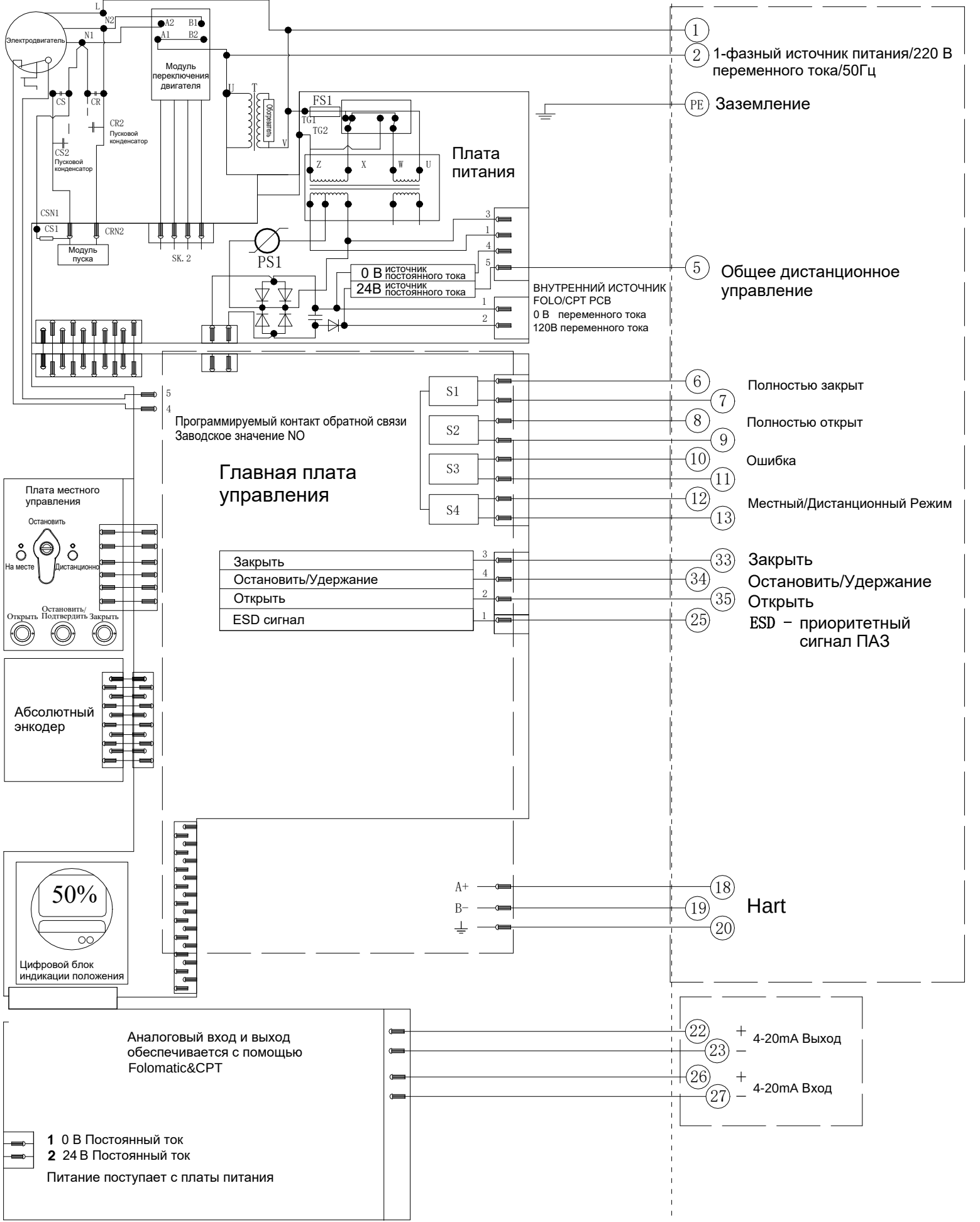
Электрическая схема №6-220-24-4-HR-1 Серия VADM
