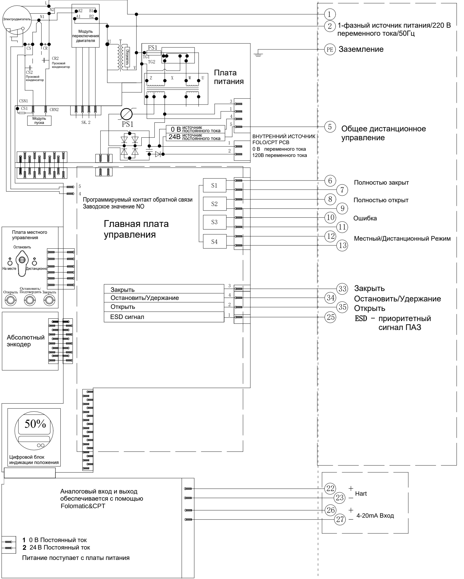
Электрическая схема №6-220-24-4-HR-2 Серия VADM
