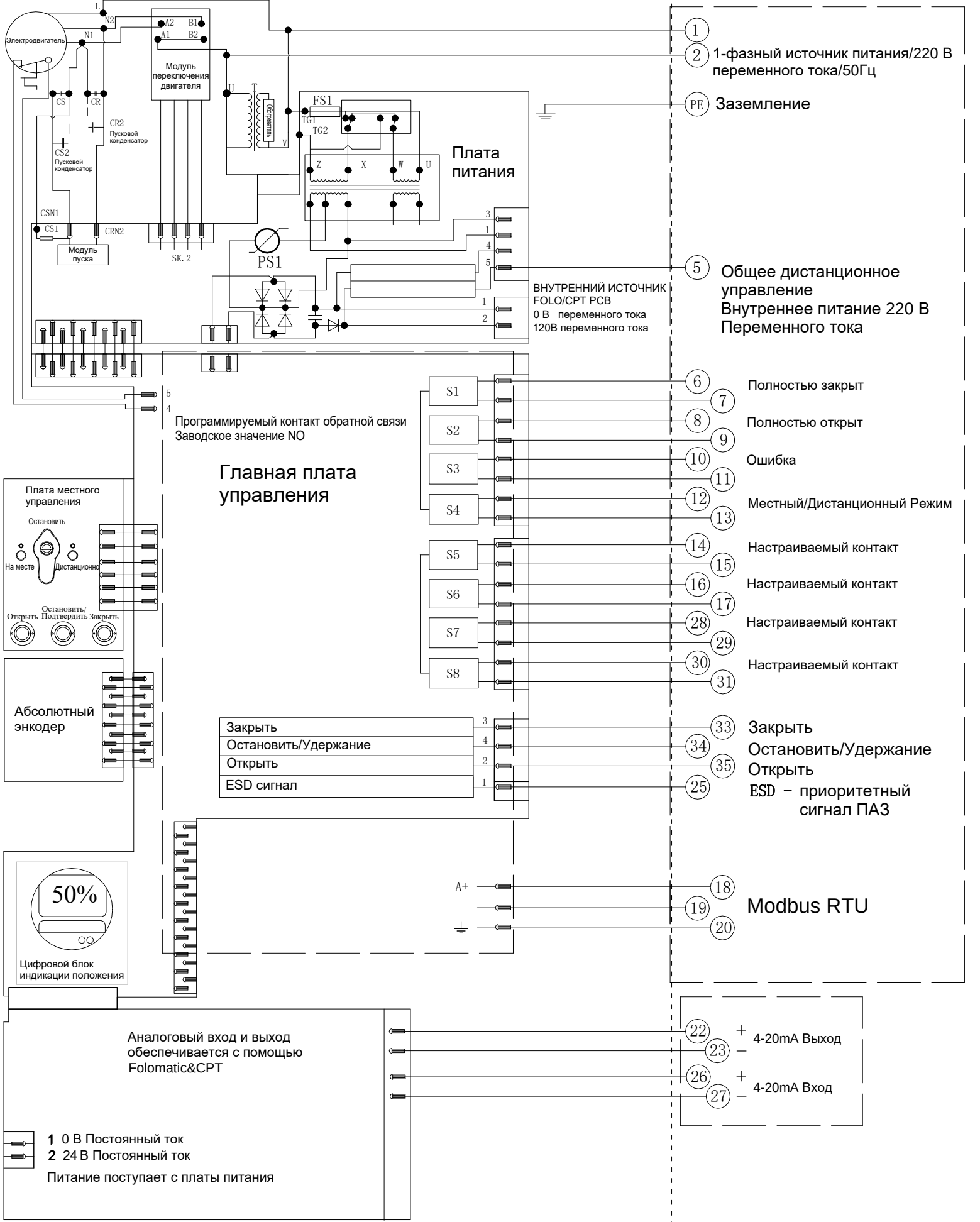
Электрическая схема №6-220-24-8-MR-1 Серия VADM
