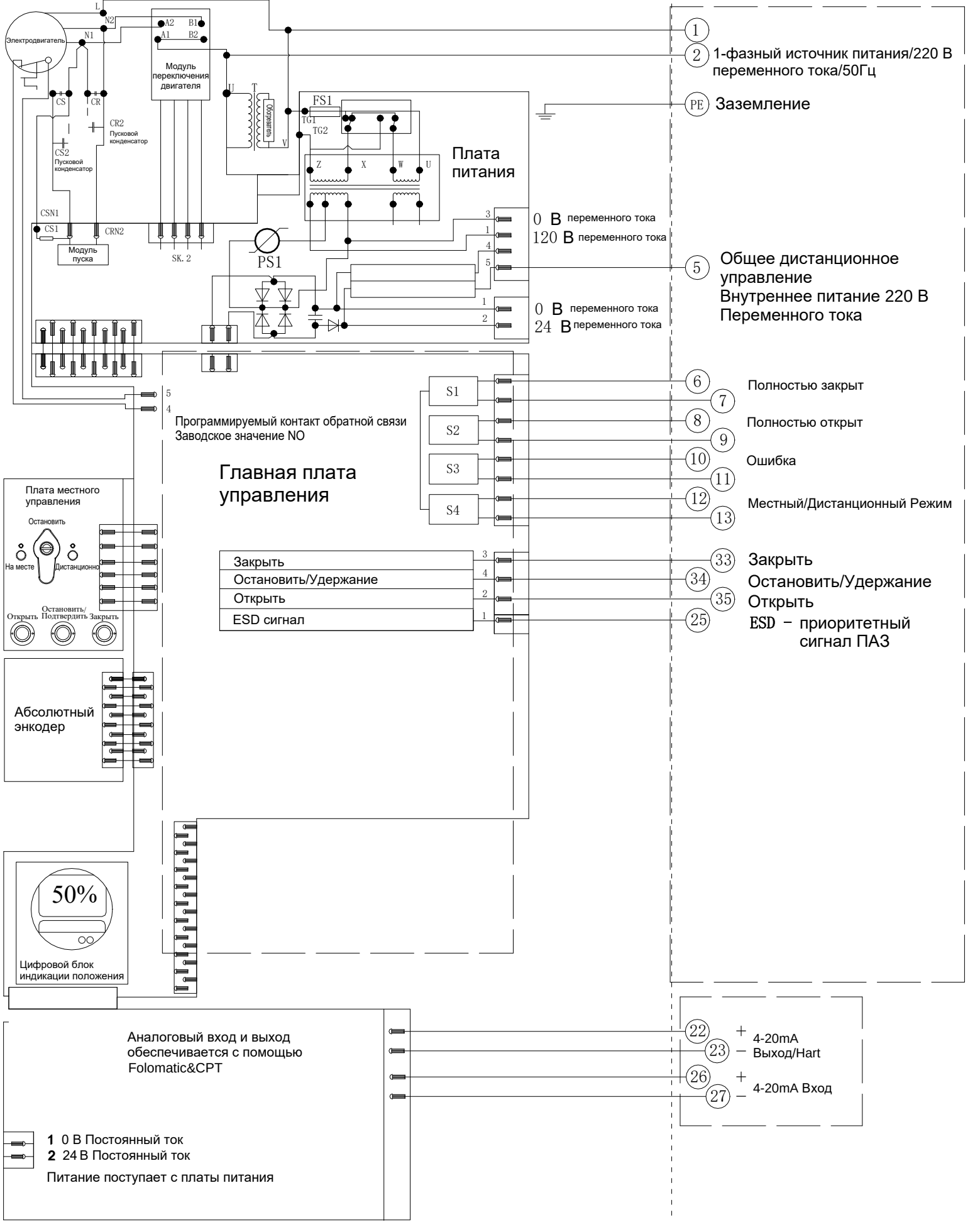
Электрическая схема №6-220-220-4-HR- 1 Серия VADM
