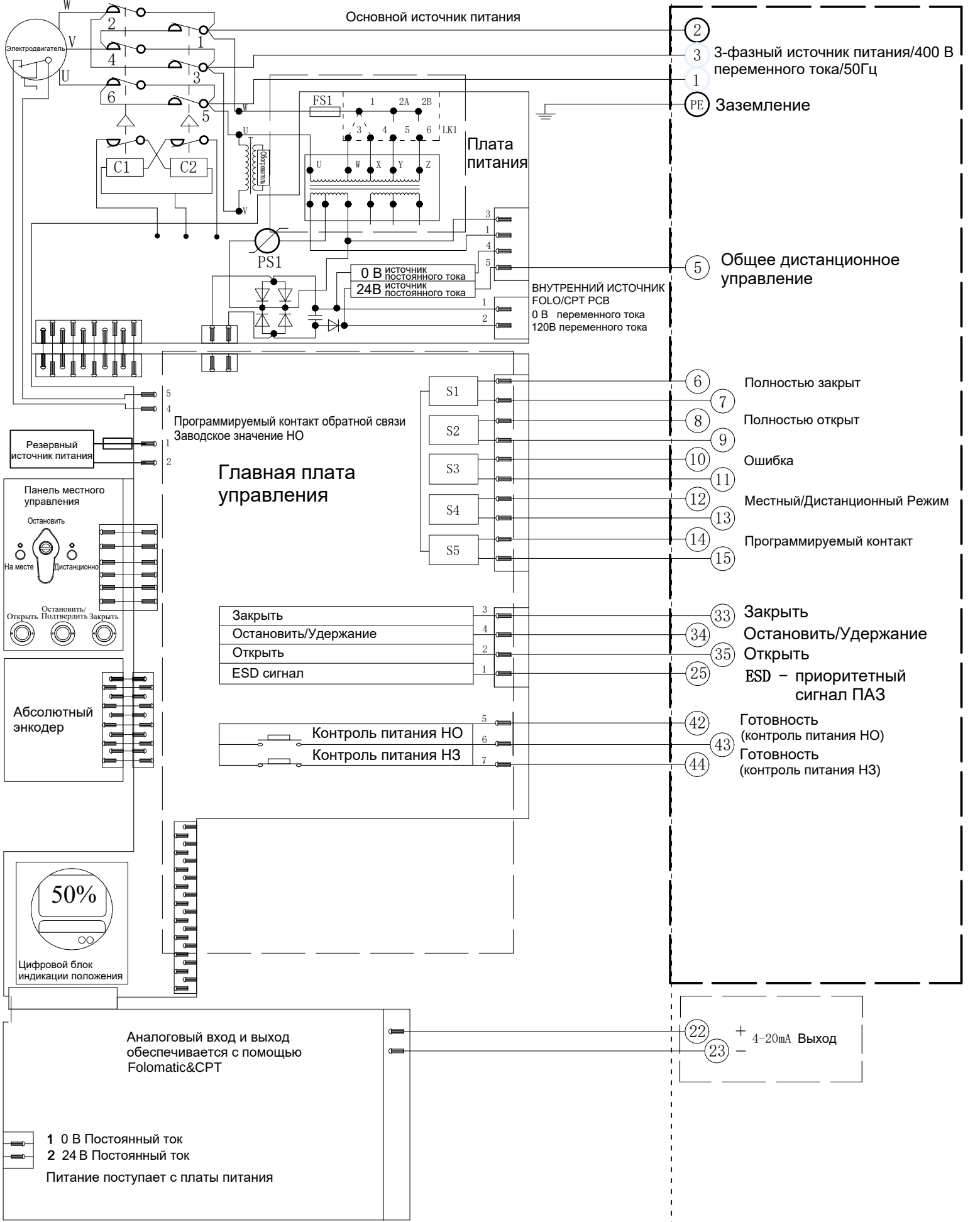
Электрическая схема №1-400В-24-6-N-3 Серия VAD
