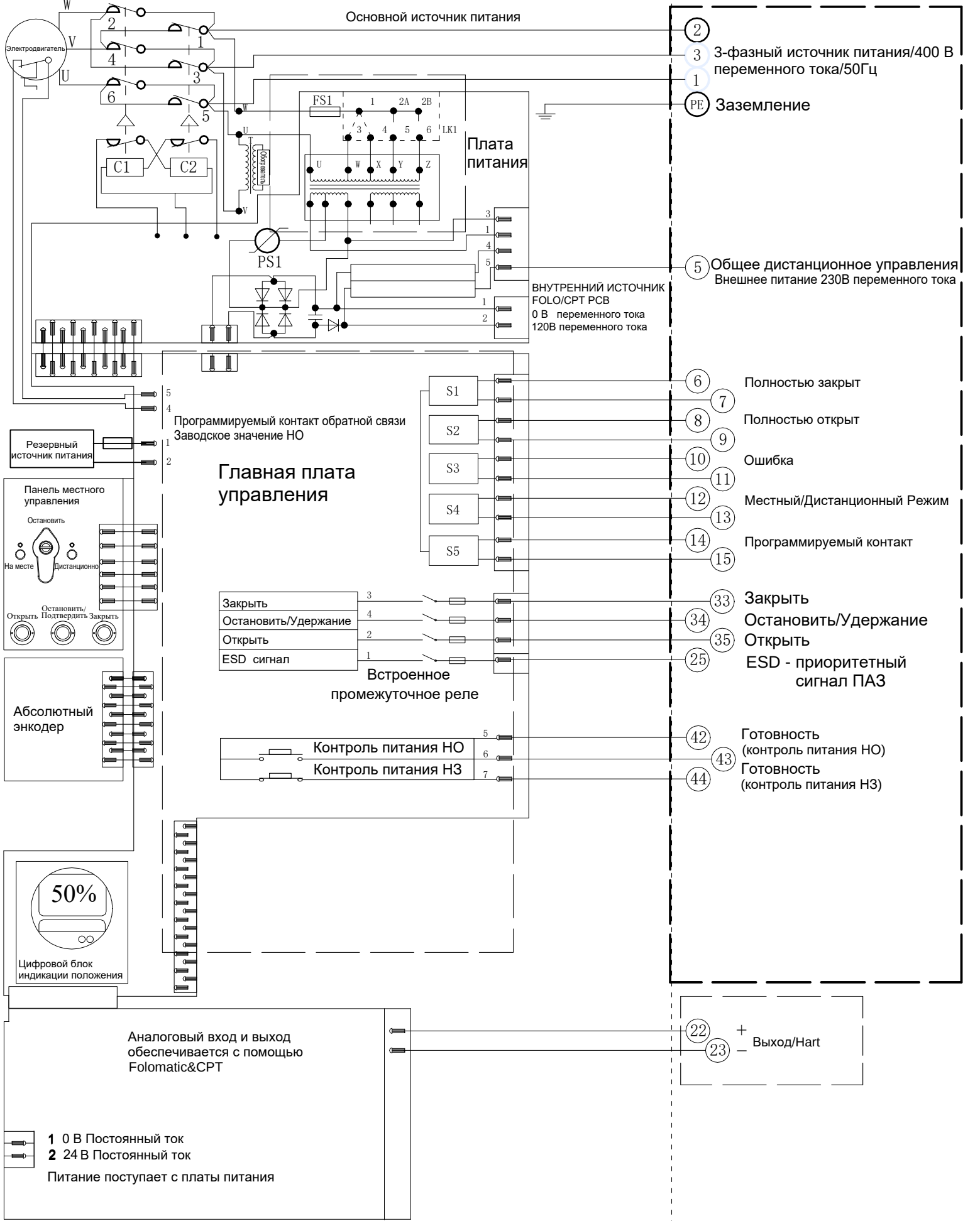
Электрическая схема №1-400В-230-6-HR-3 Серия VAD
