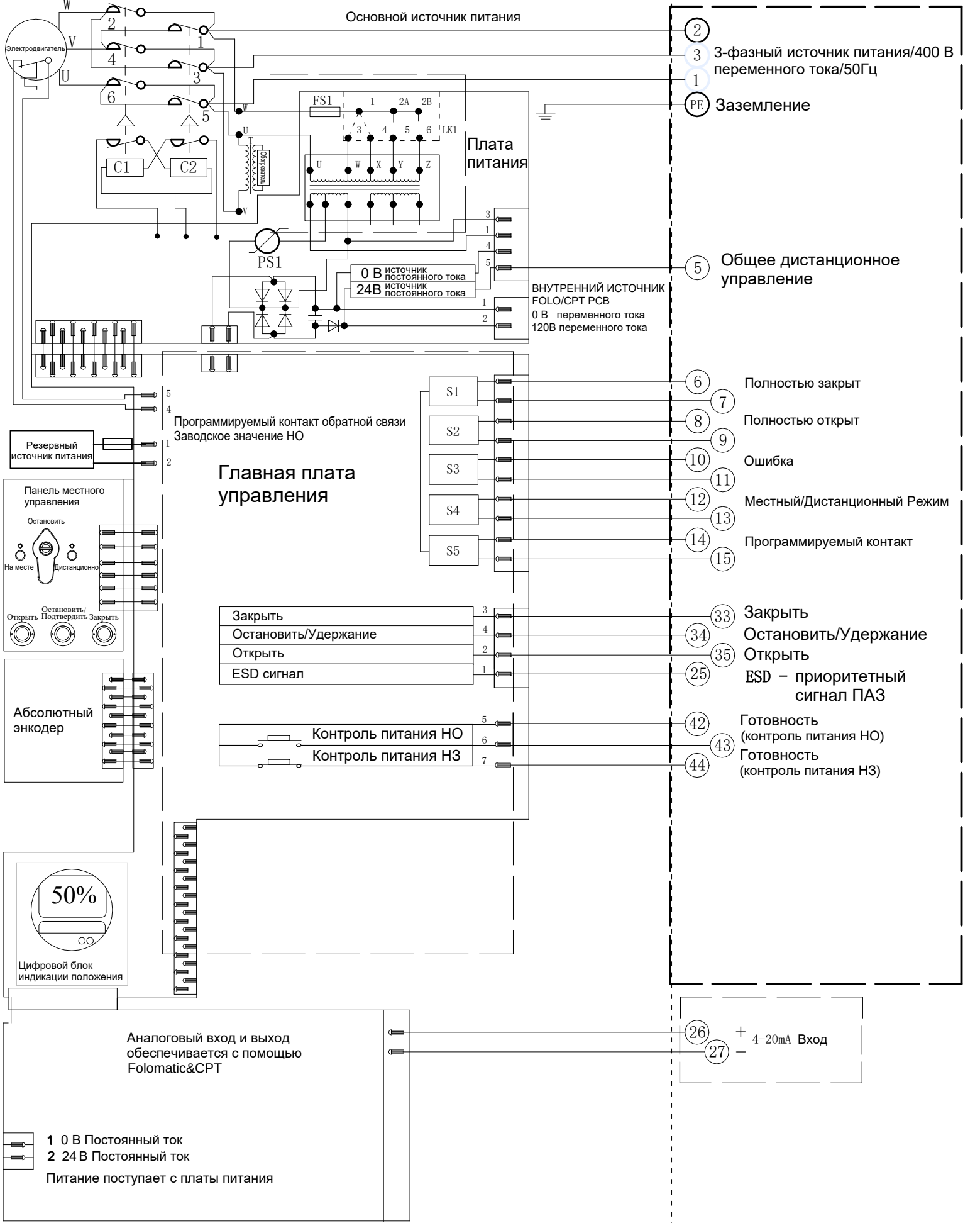
Электрическая схема №1-400В-24-6-N-2 Серия VAD
