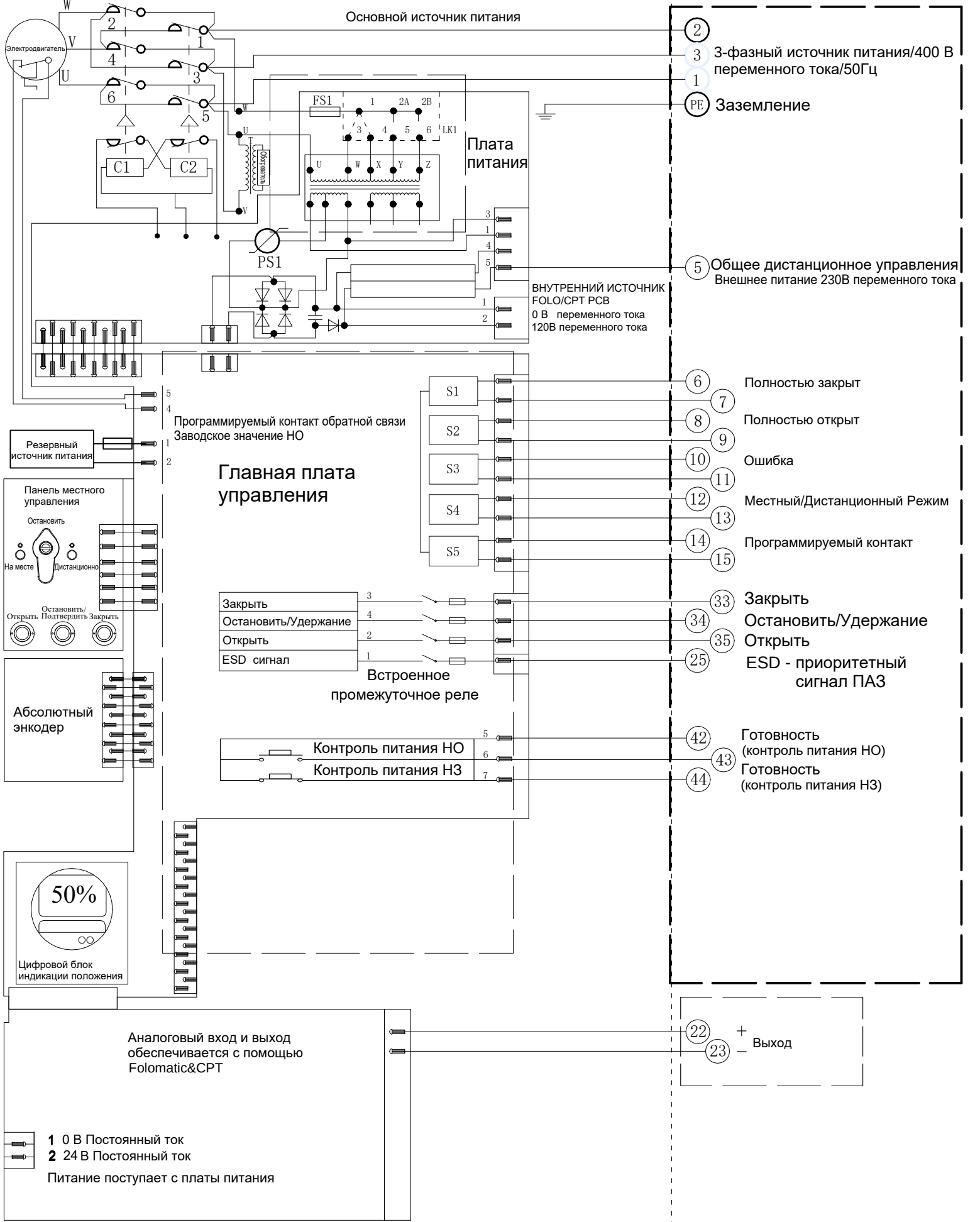
Электрическая схема №1-400В-230-6-N-3 Серия VAD
