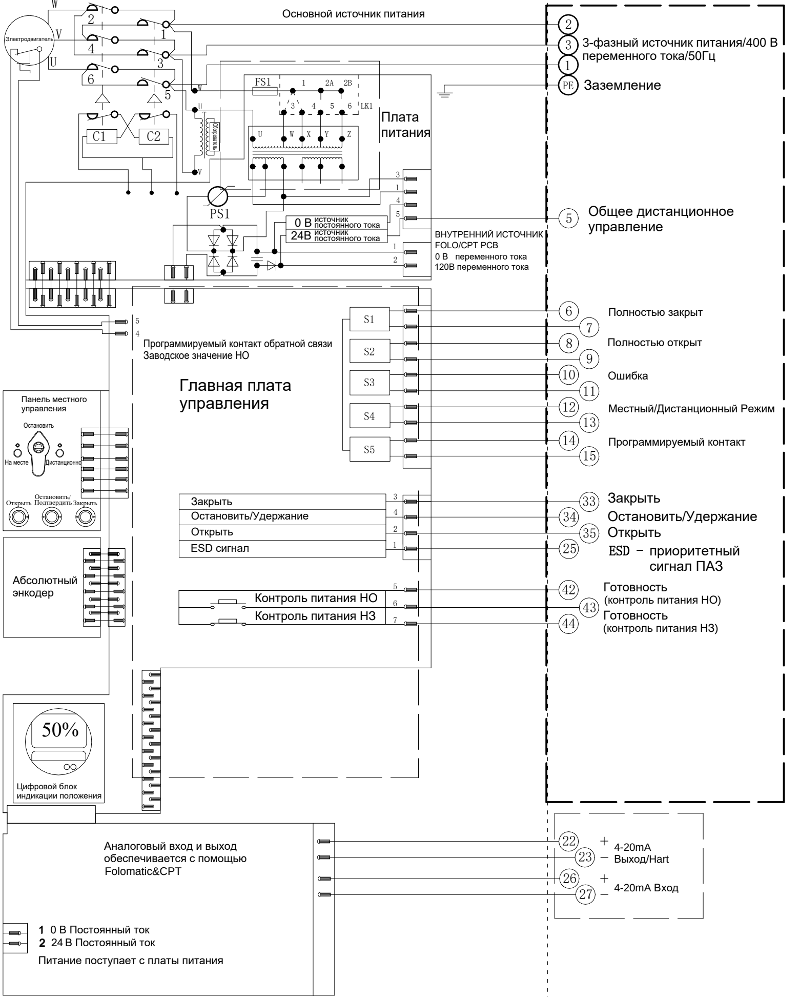
Электрическая схема №1-400-24-6-HR- 1 Серия VAD
