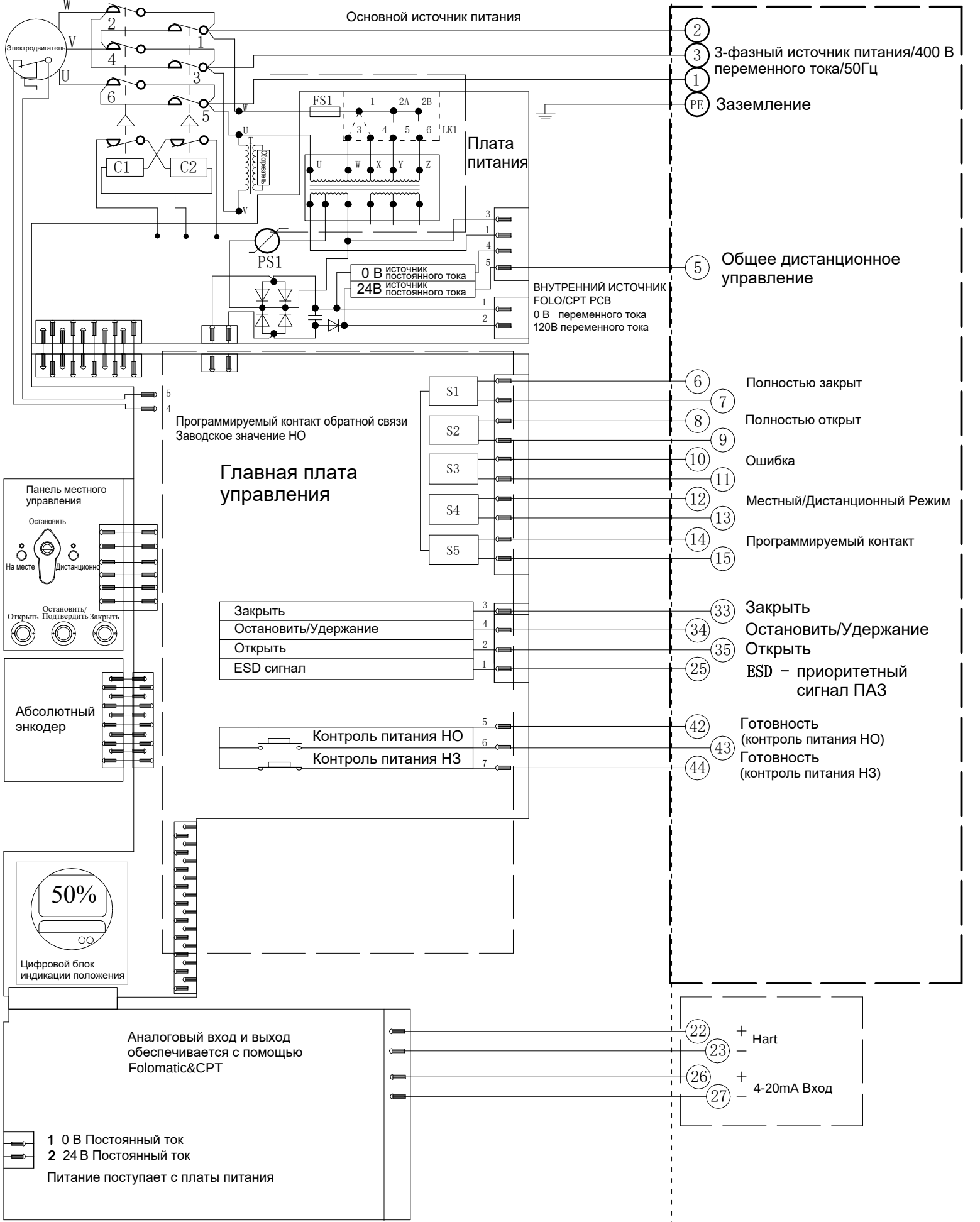
Электрическая схема №1-400-24-6-HR-2 Серия VAD
