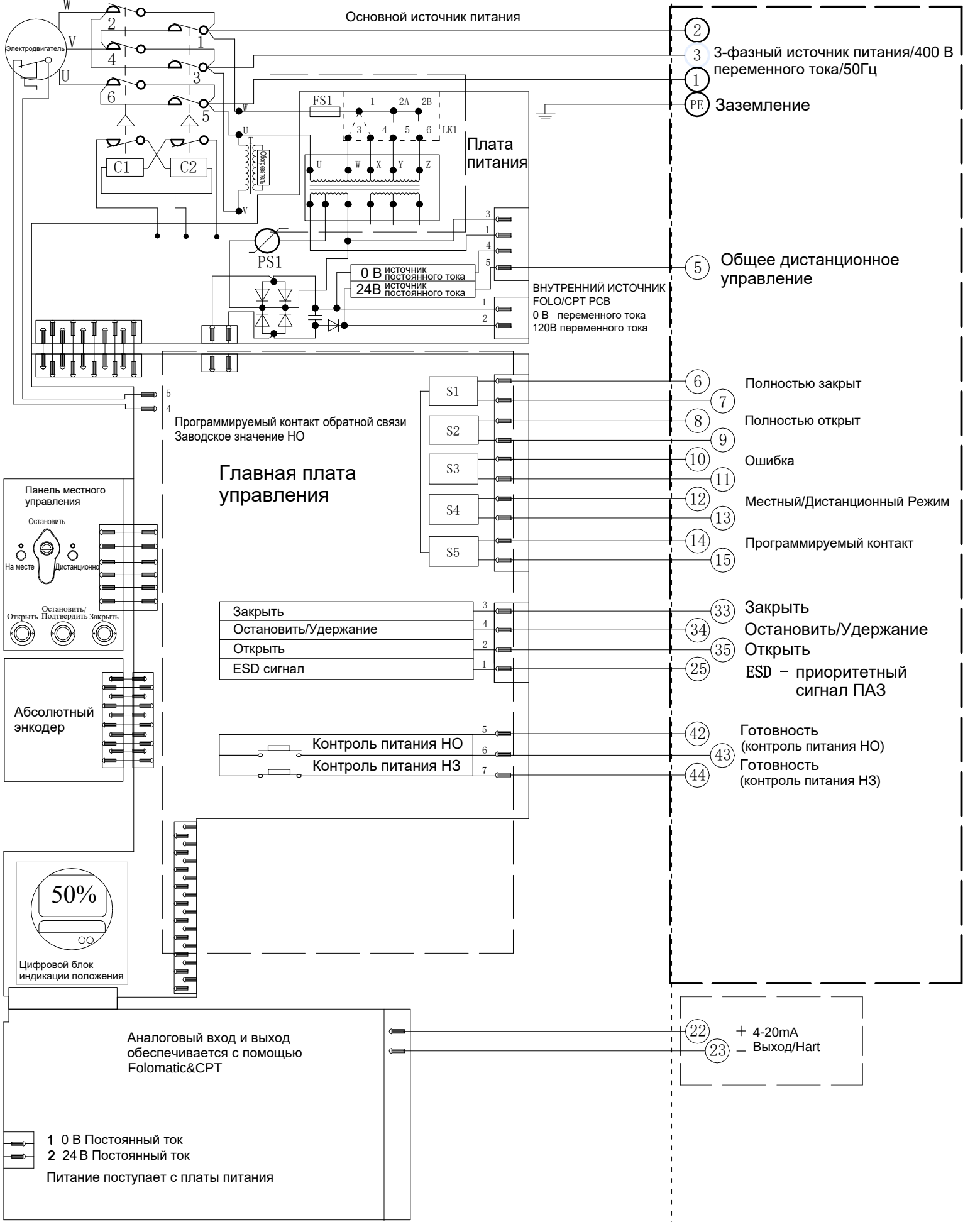
Электрическая схема №1-400-24-6-HR-3 Серия VAD
