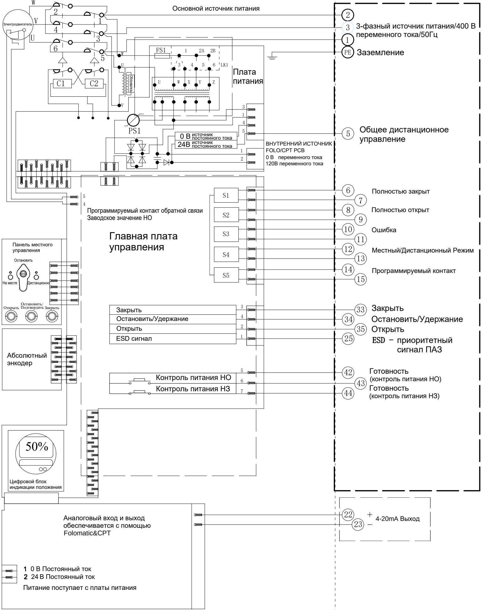
Электрическая схема №1-400-24-6-N-3 Серия VAD
