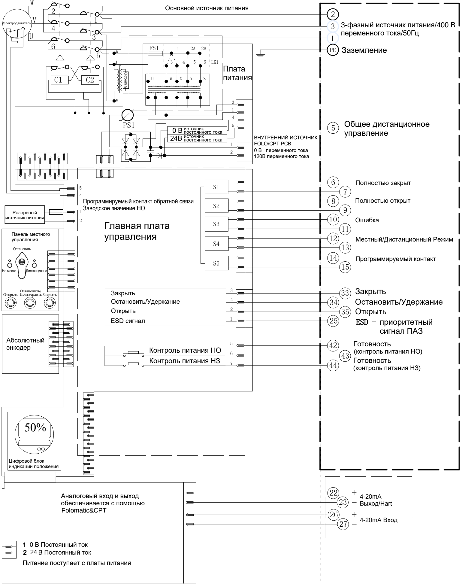
Электрическая схема №1-400В-24-6-HR-1 Серия VAD
