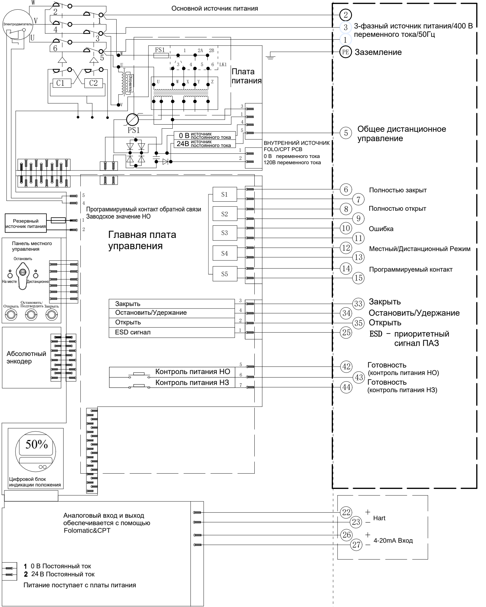
Электрическая схема №1-400В-24-6-HR-2 Серия VAD
