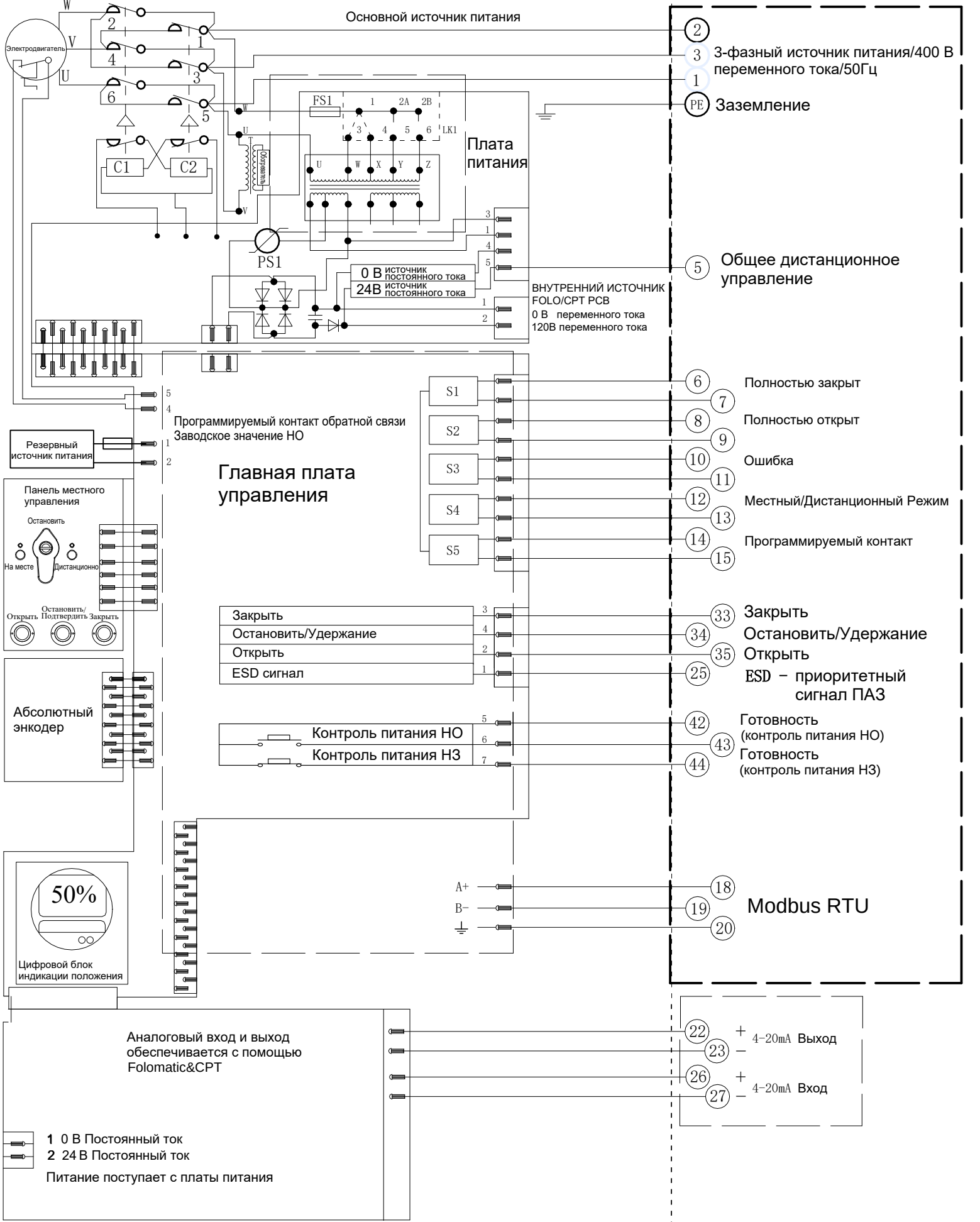
Электрическая схема №1-400B-24-6-MR-1 Серия VAD
