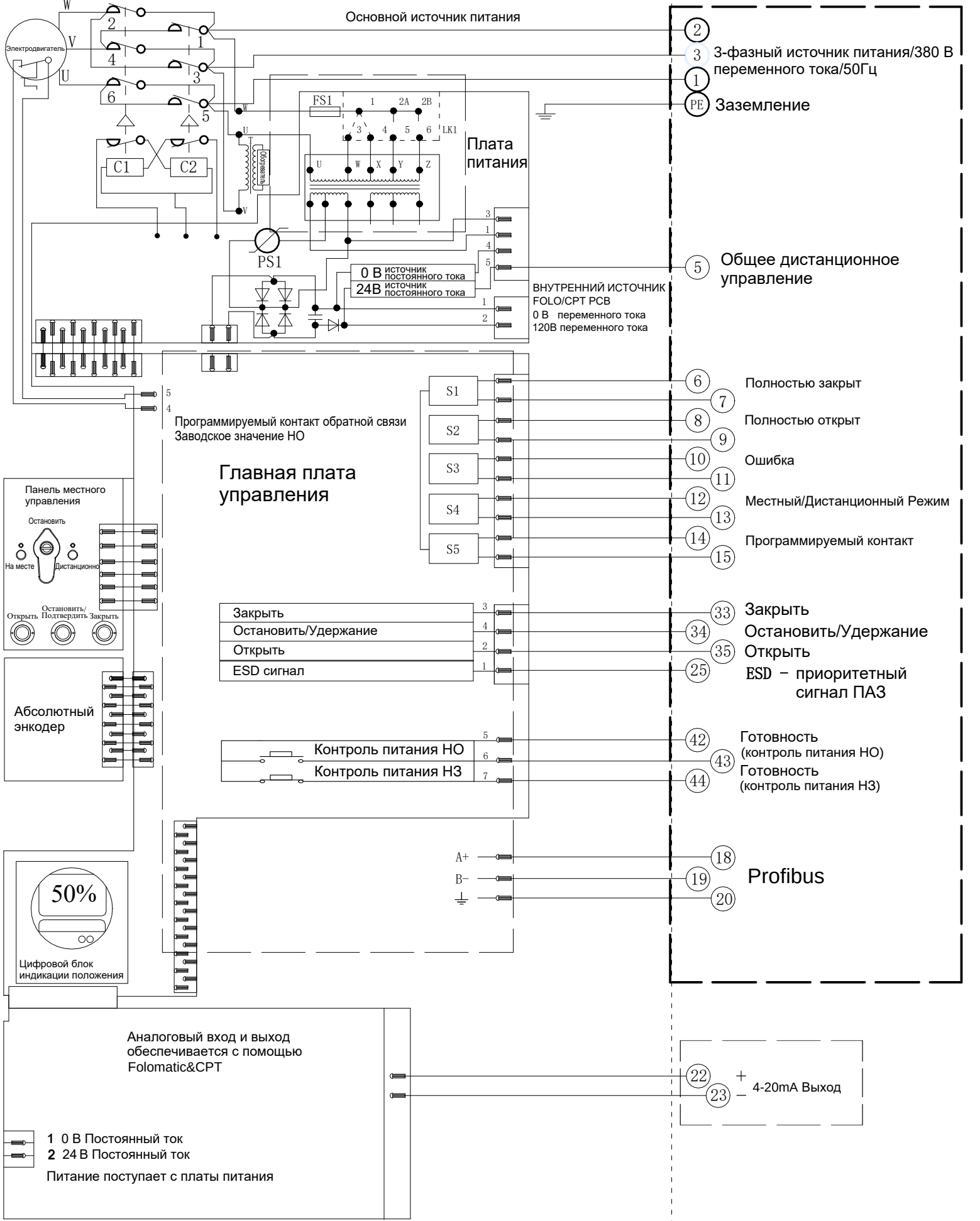
Электрическая схема №1-380-24-6-PR-3 Серия VAD
