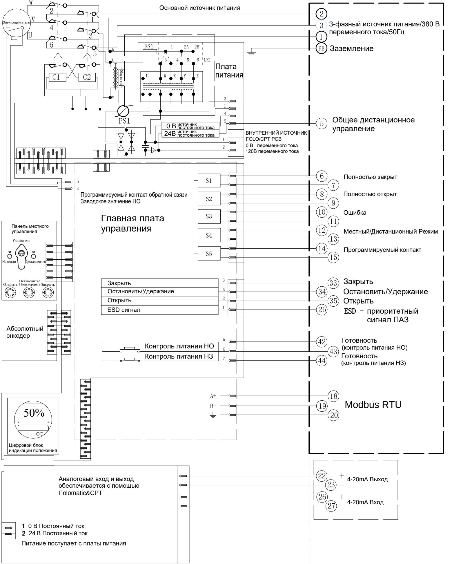
Электрическая схема №1-380-24-6-MR-1 Серия VAD
