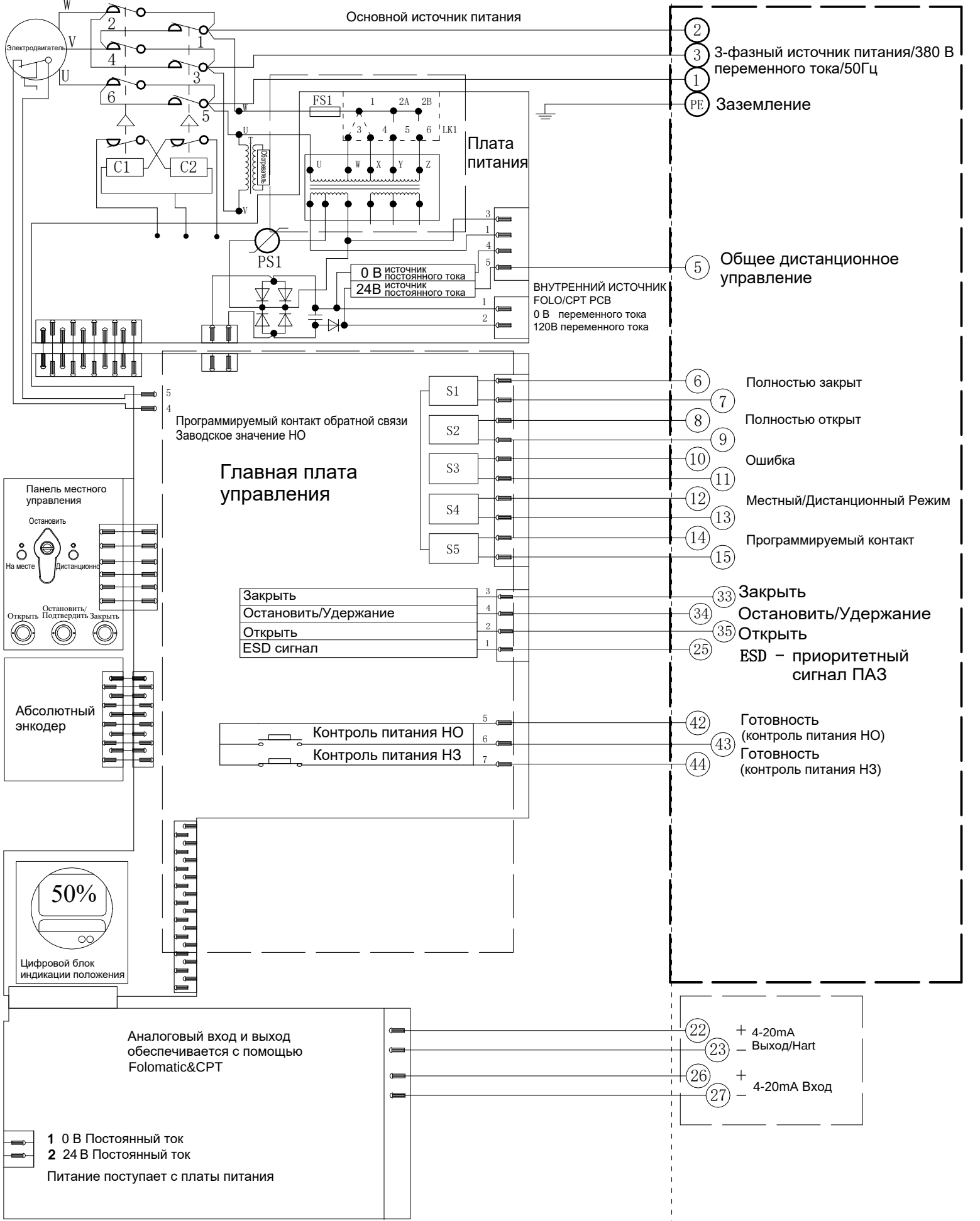
Электрическая схема №1-380-24-6-HR-1 Серия VAD
