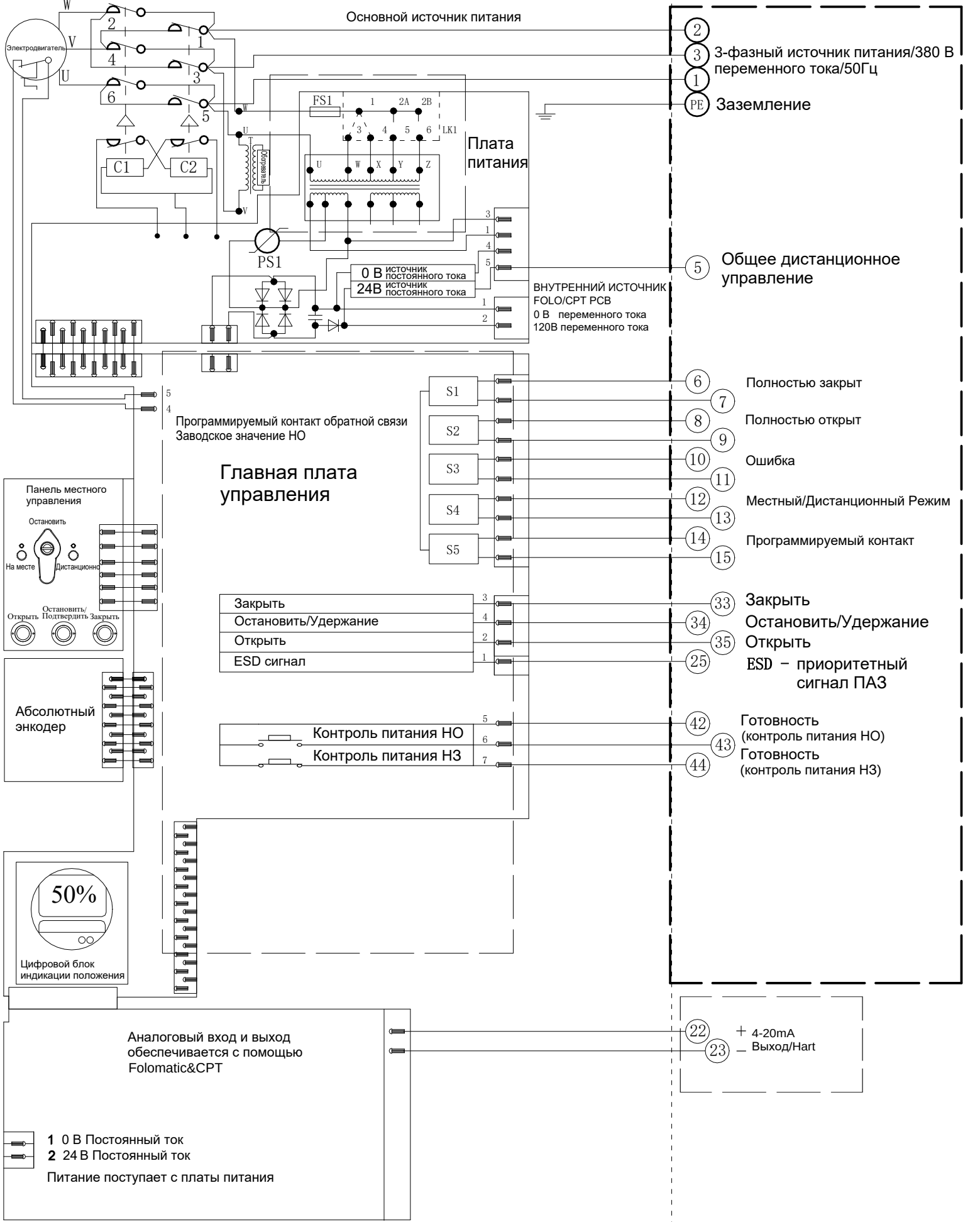
Электрическая схема №1-380-24-6-HR-3 Серия VAD
