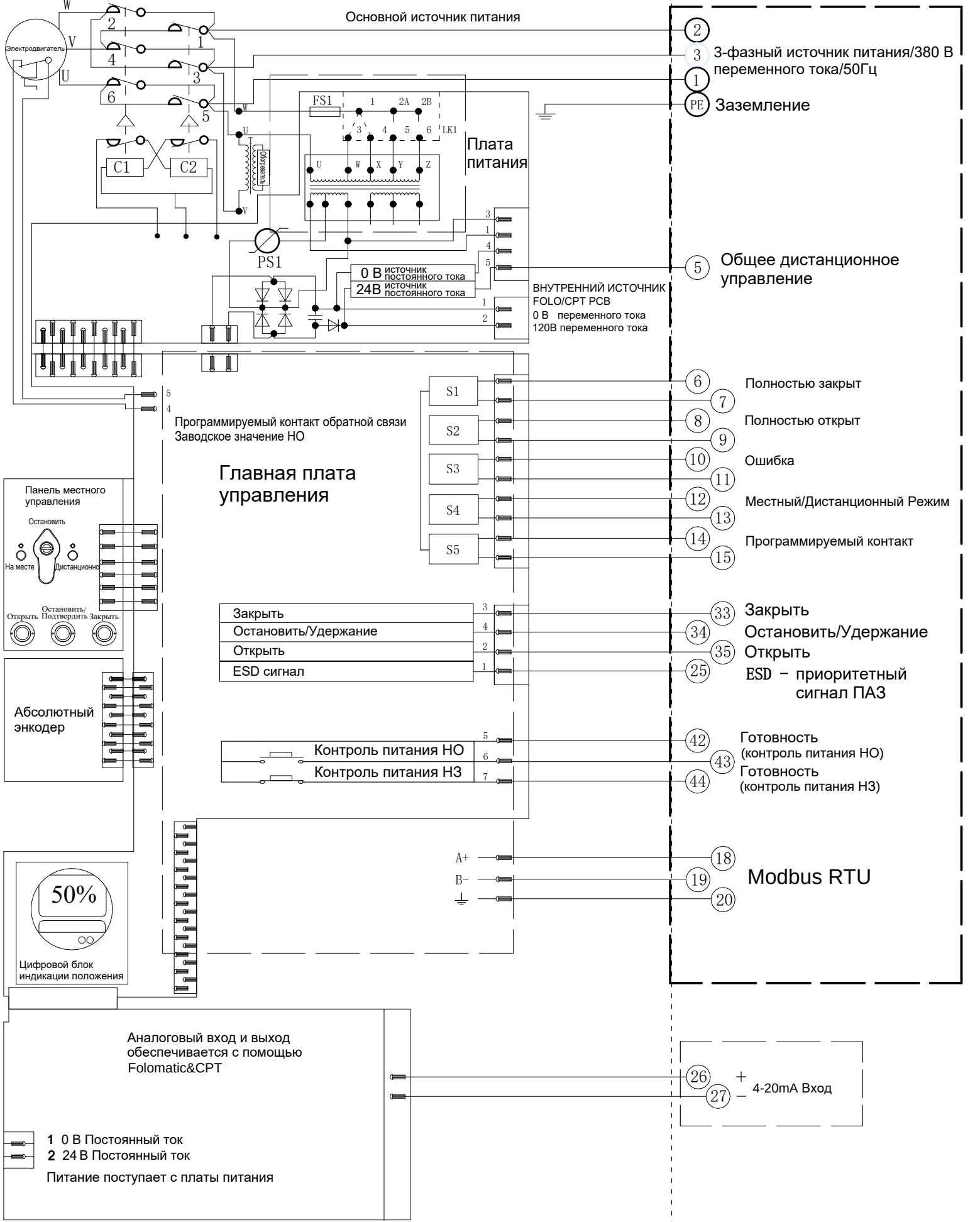
Электрическая схема №1-380-24-6-MR-2 Серия VAD
