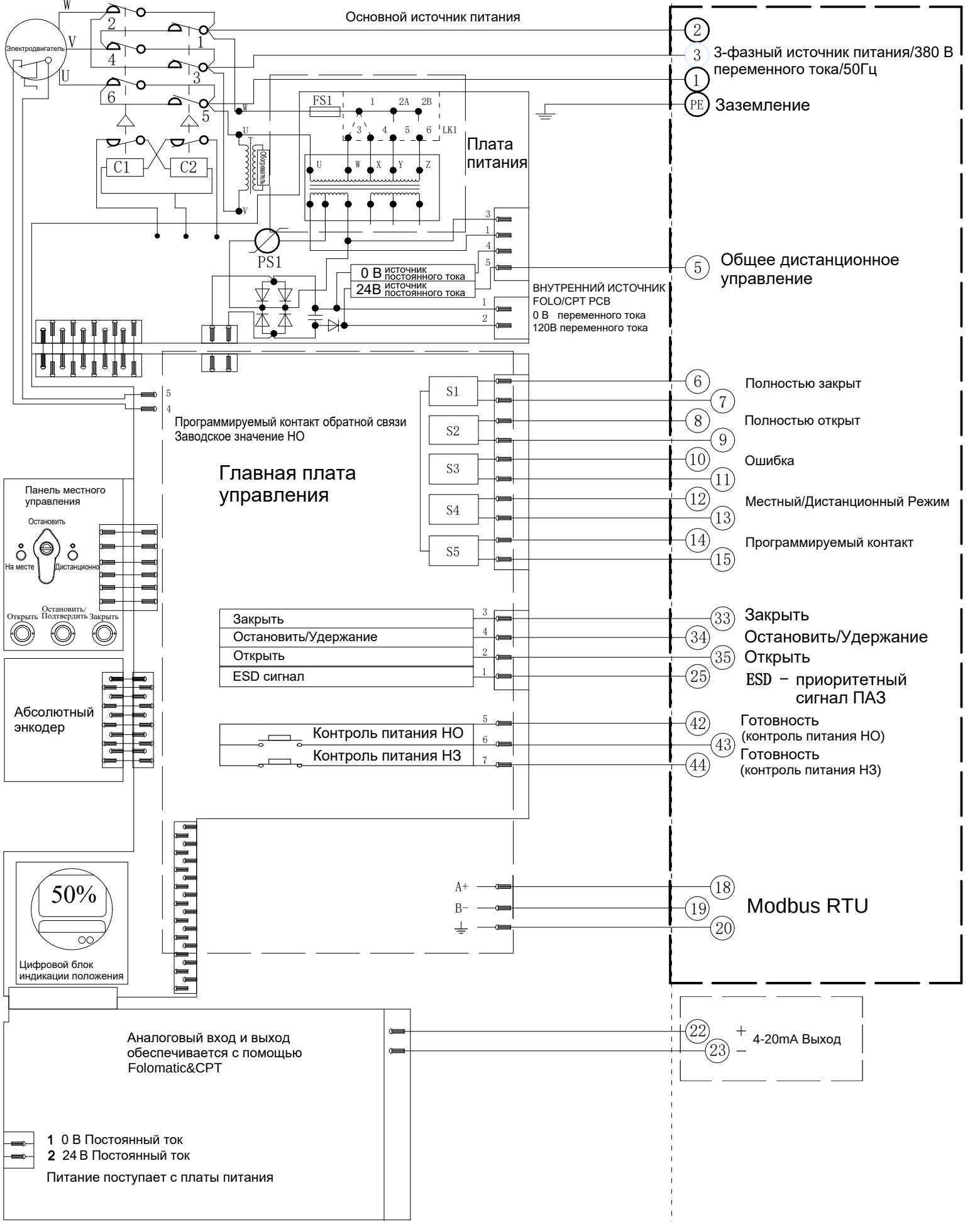
Электрическая схема №1-380-24-6-MR-3 Серия VAD
