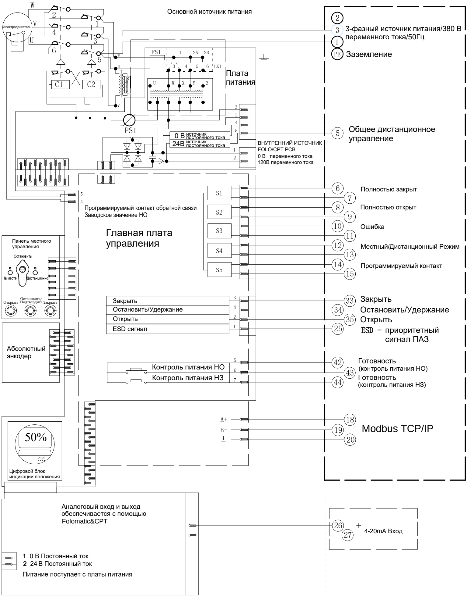
Электрическая схема №1-380-24-6-MT-2 Серия VAD
