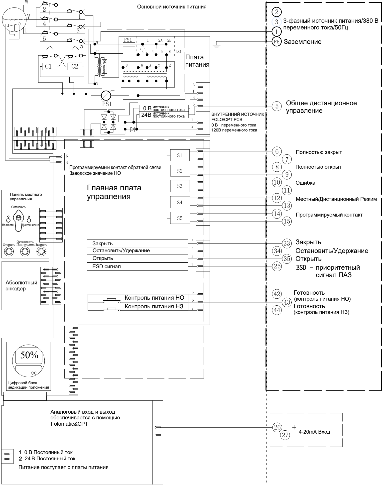
Электрическая схема №1-380-24-6-N-2 Серия VAD
