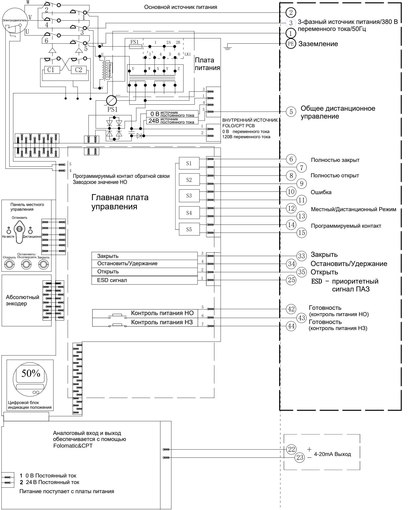
Электрическая схема №1-380-24-6-N-3 Серия VAD
