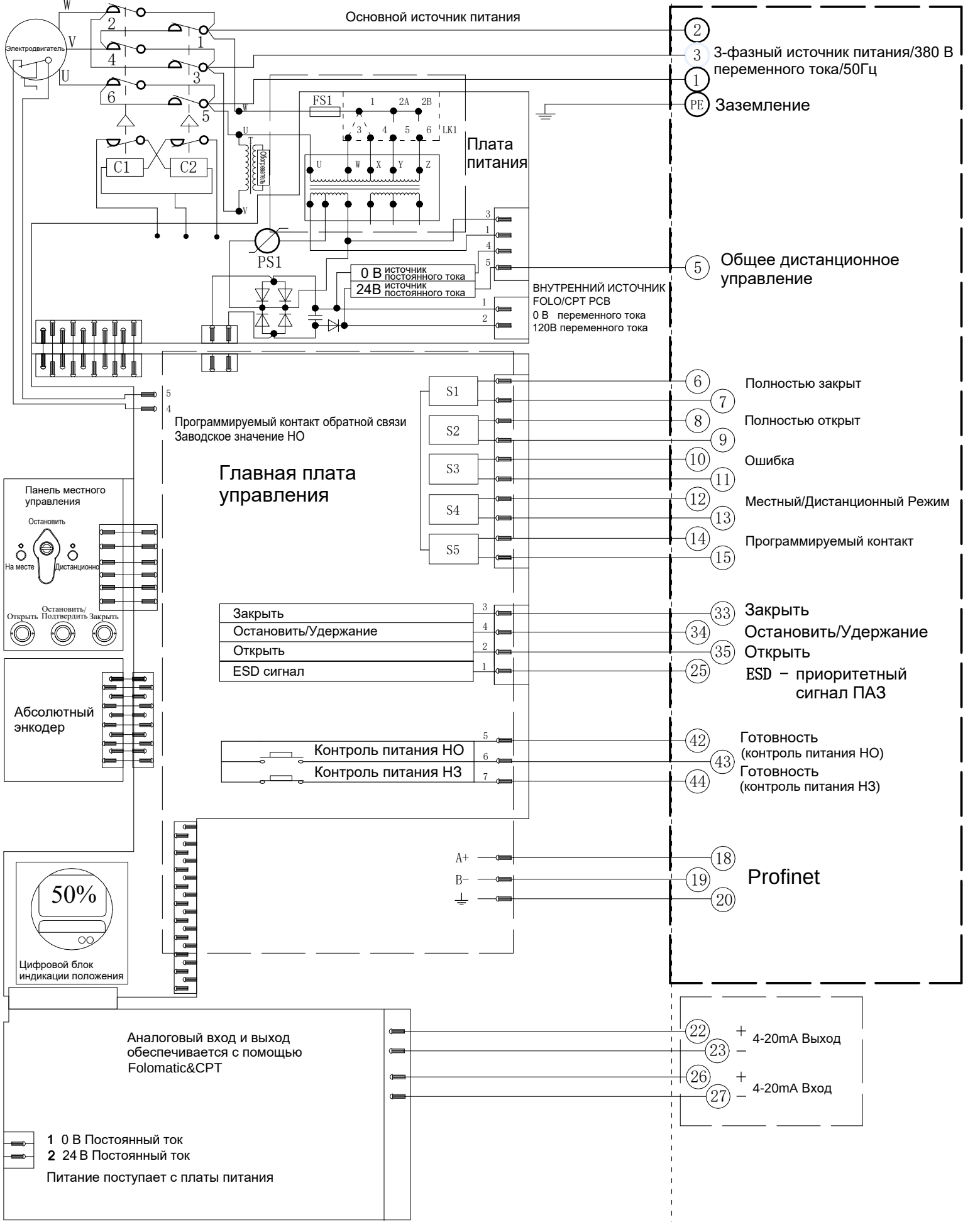
Электрическая схема №1-380-24-6-PN-1 Серия VAD
