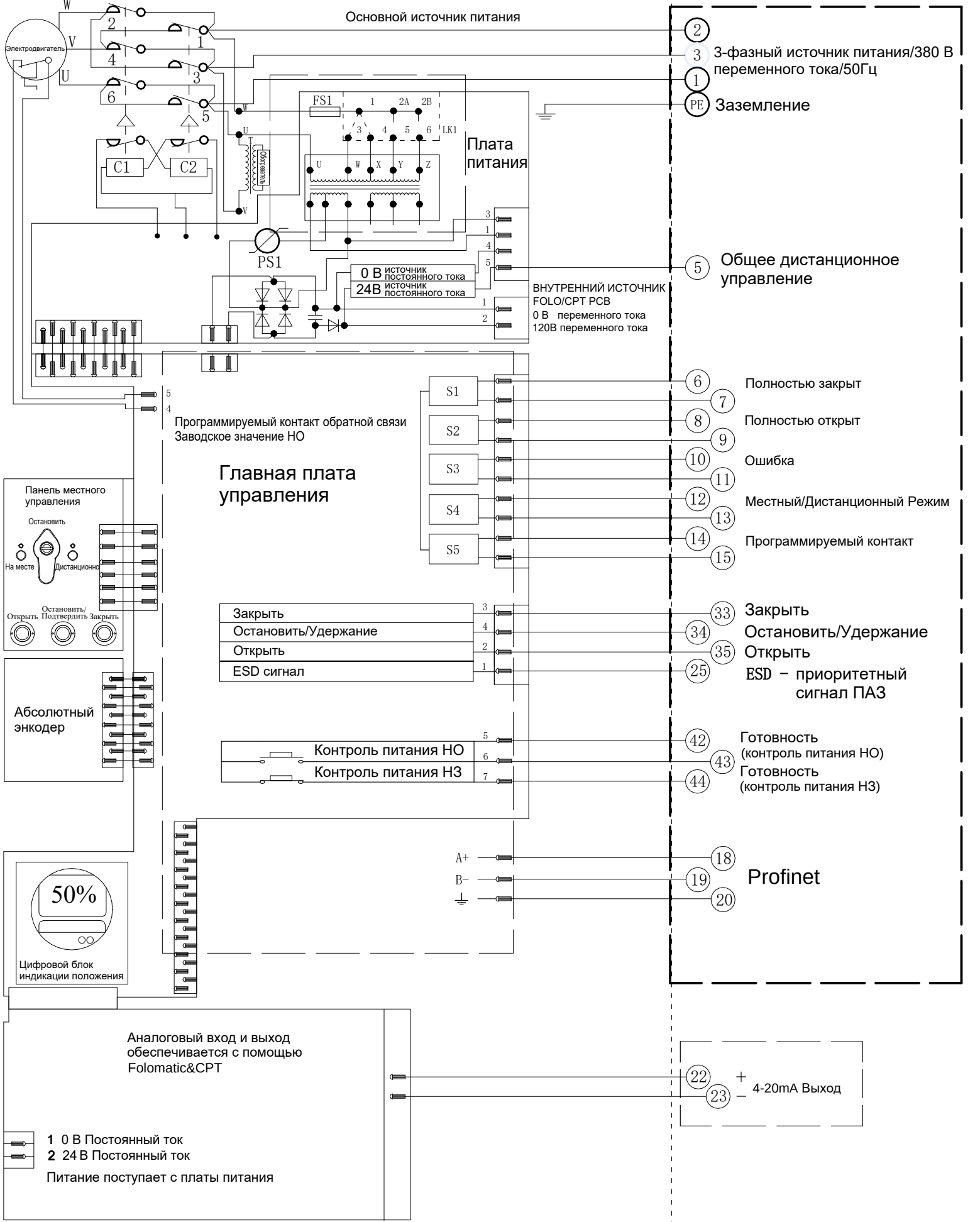
Электрическая схема №1-380-24-6-PN-3 Серия VAD
