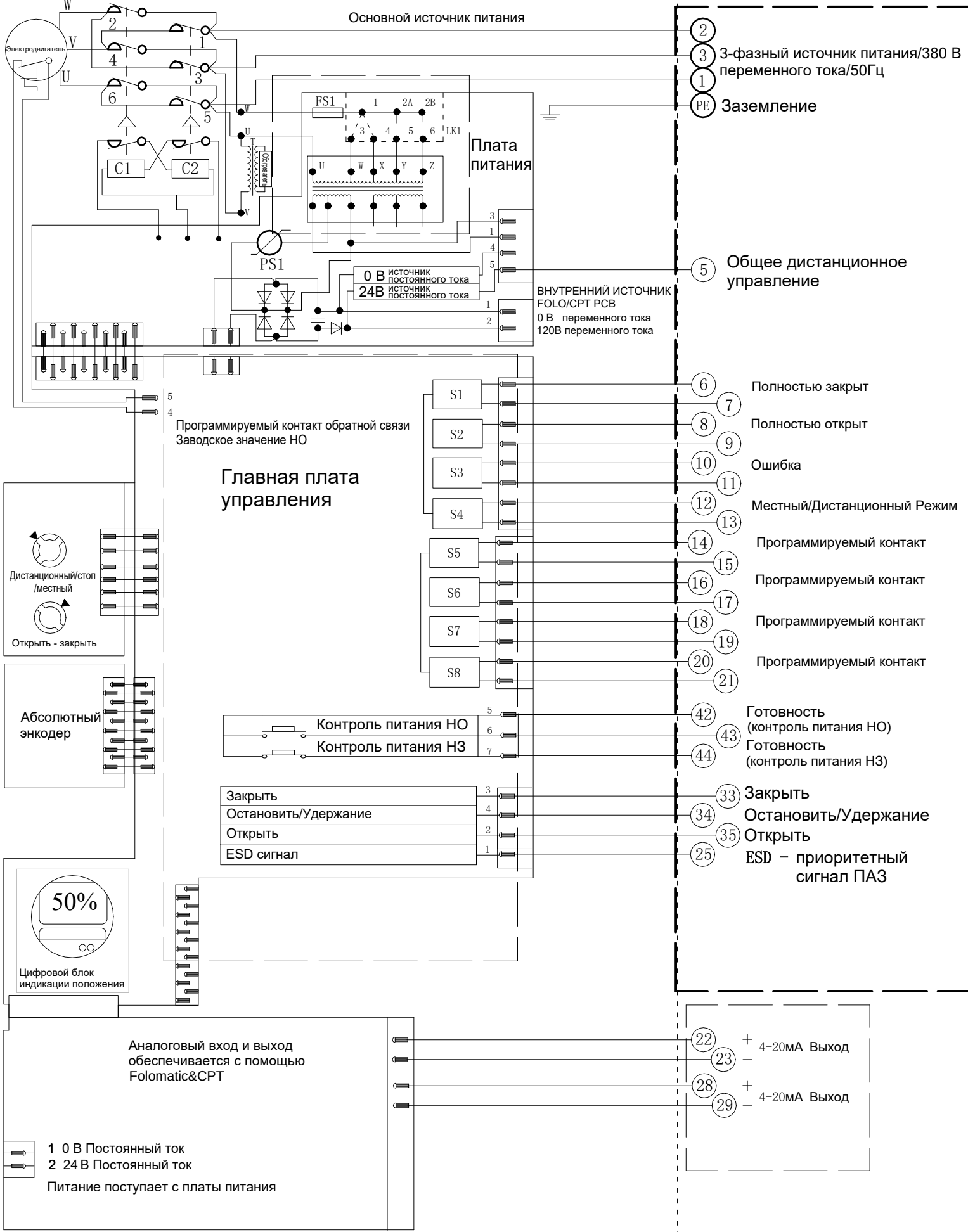
Электрическая схема №1-380-24-9-N-8 Серия VAD
