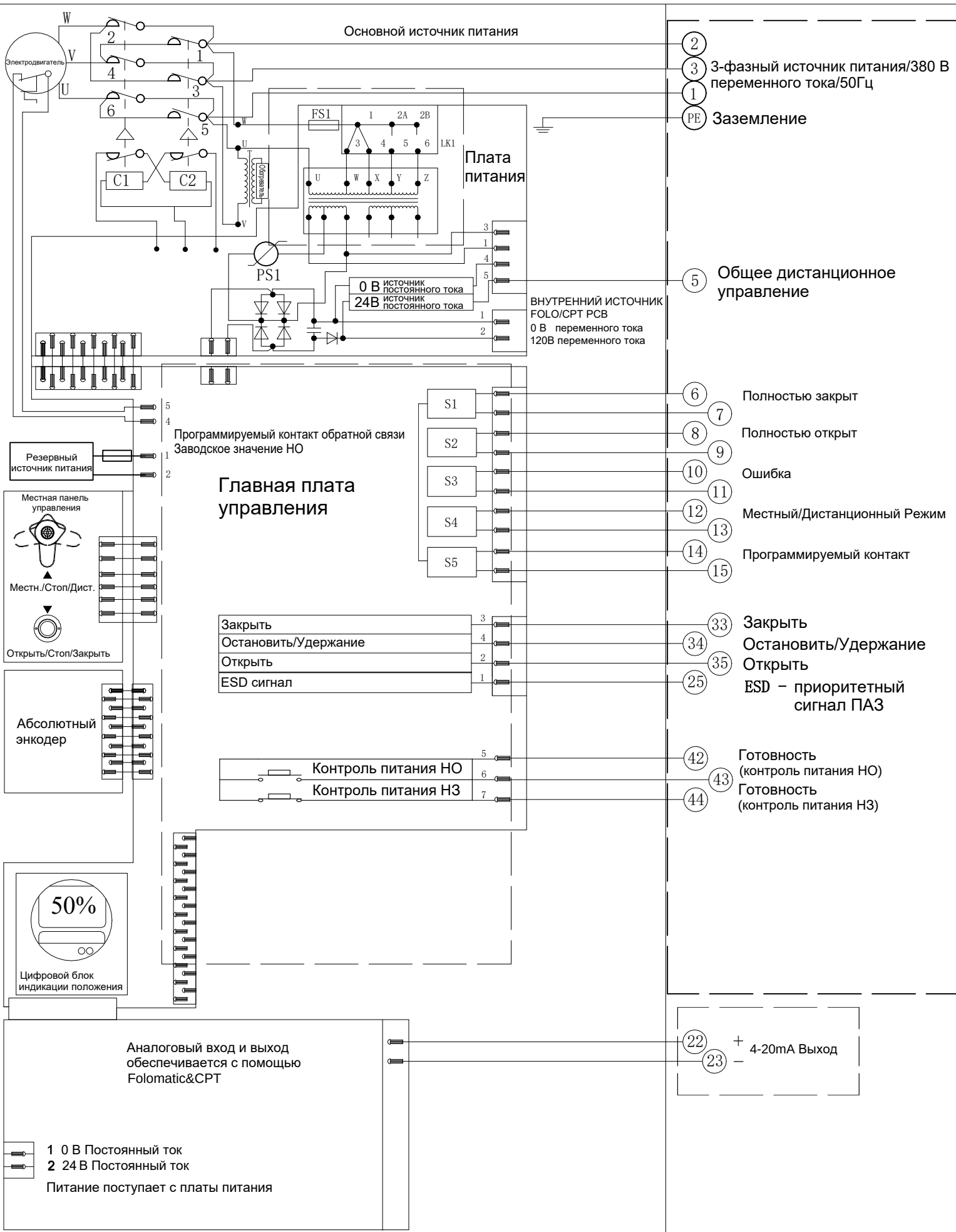
Электрическая схема №1-380В-24-6-N-3 Серия VAD
