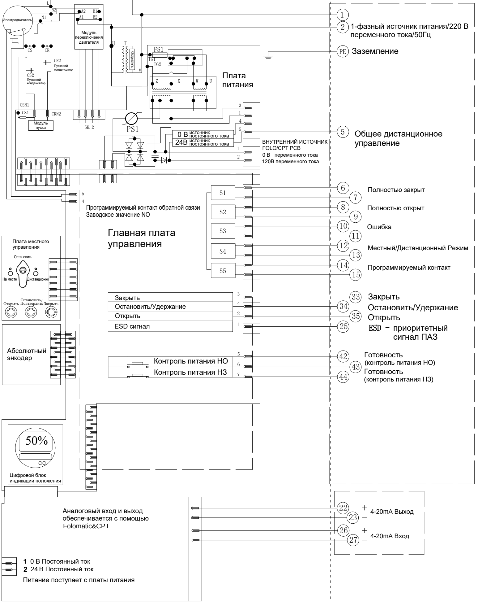
Электрическая схема №1-220-24-6-N-1 Серия VAD
