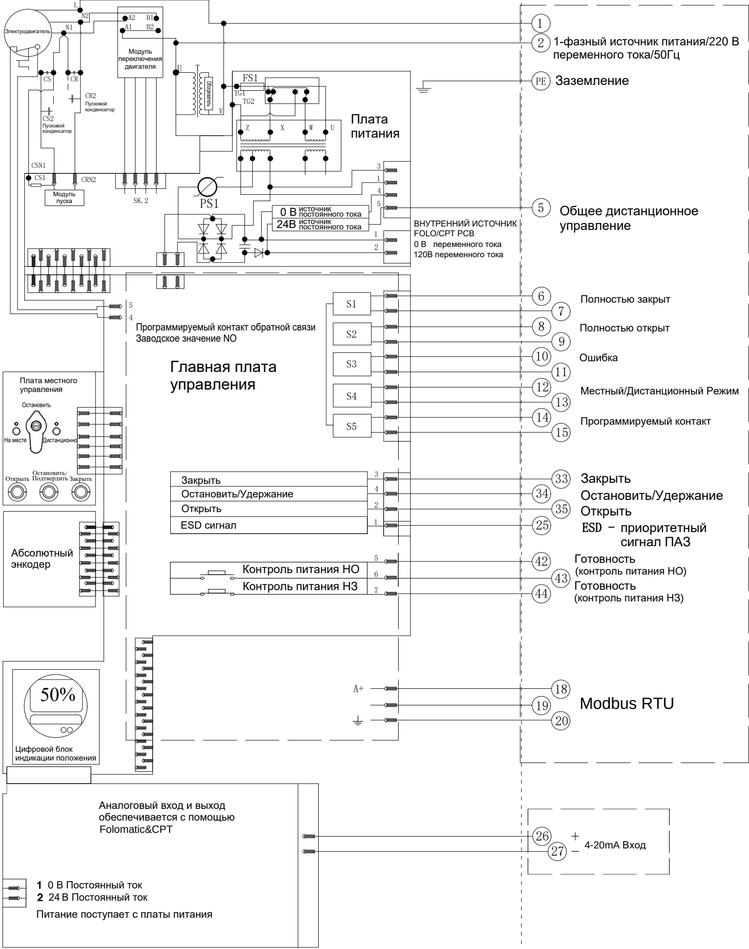
Электрическая схема №1-220-24-6-MR-2 Серия VAD
