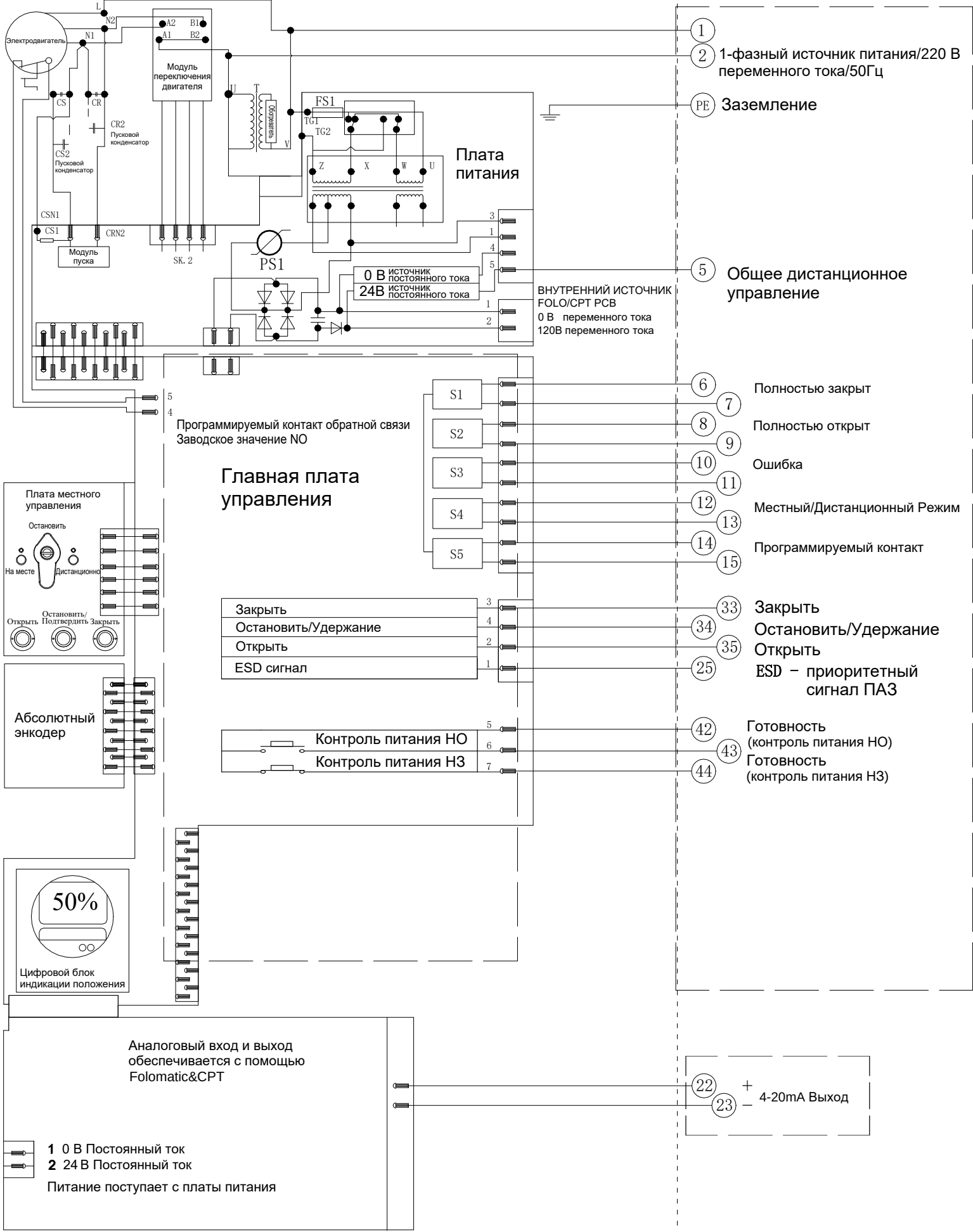
Электрическая схема №1-220-24-6-N-3 Серия VAD
