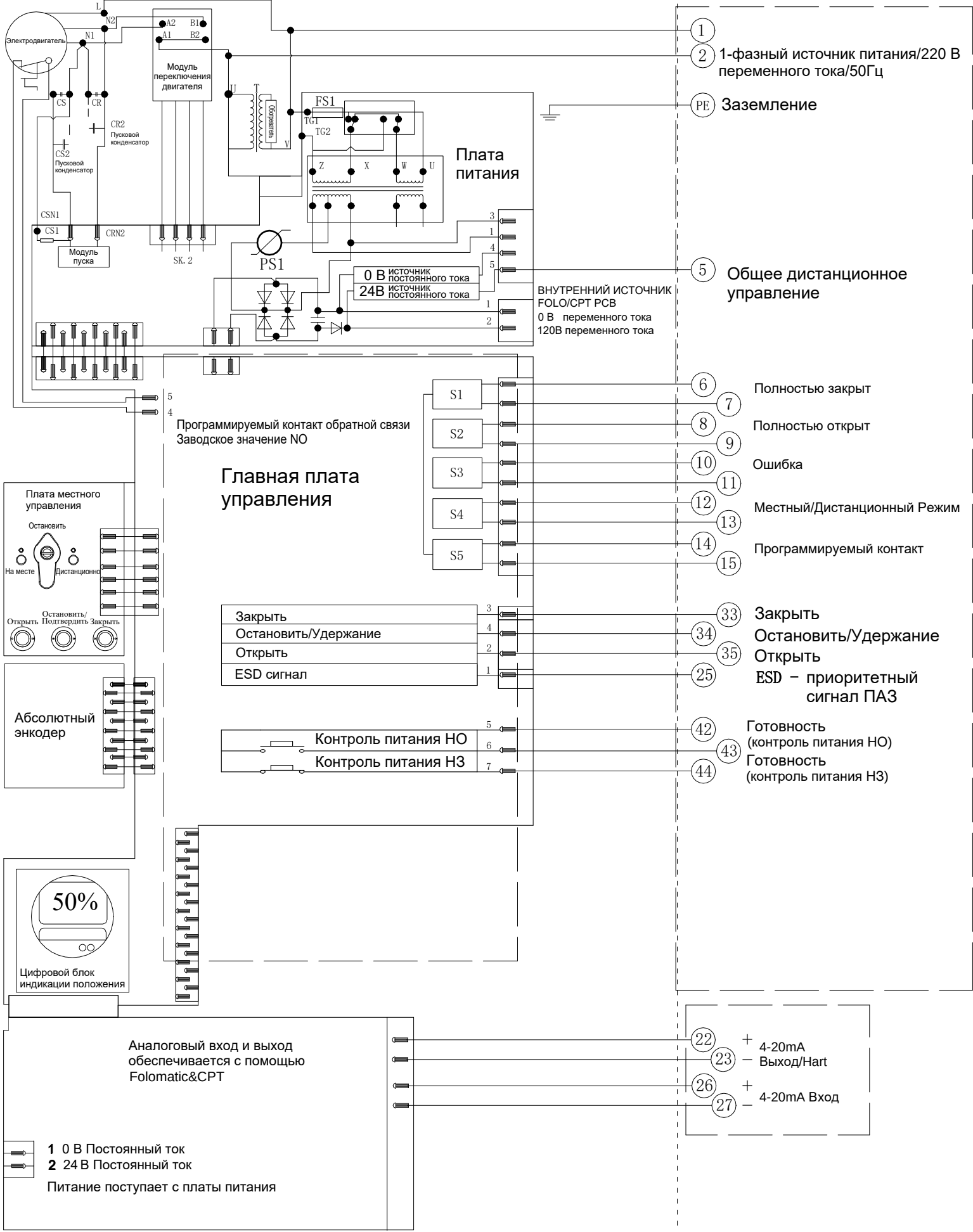
Электрическая схема №1-220-24-6-HR- 1 Серия VAD
