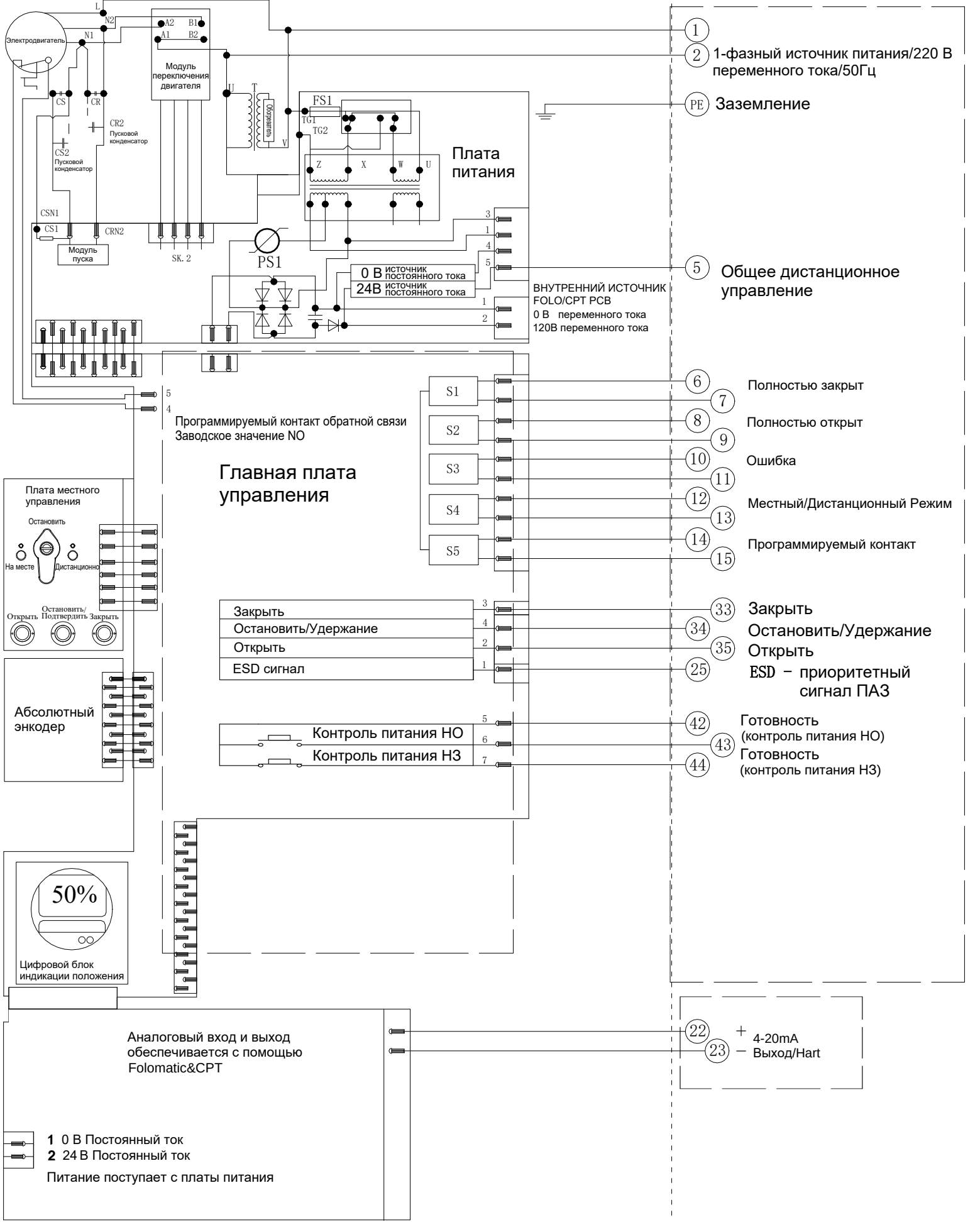
Электрическая схема №1-220-24-6-HR-3 Серия VAD
