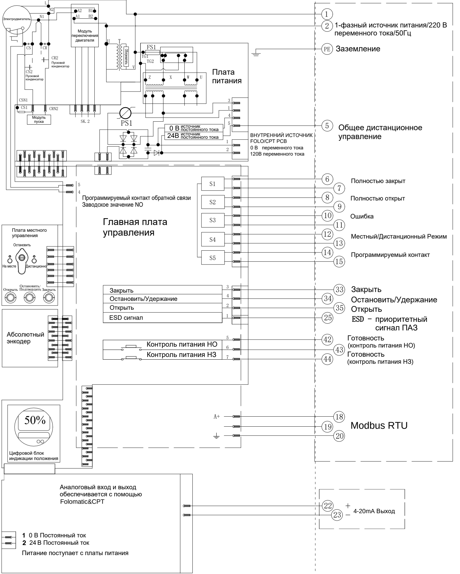
Электрическая схема №1-220-24-6-MR-3 Серия VAD
