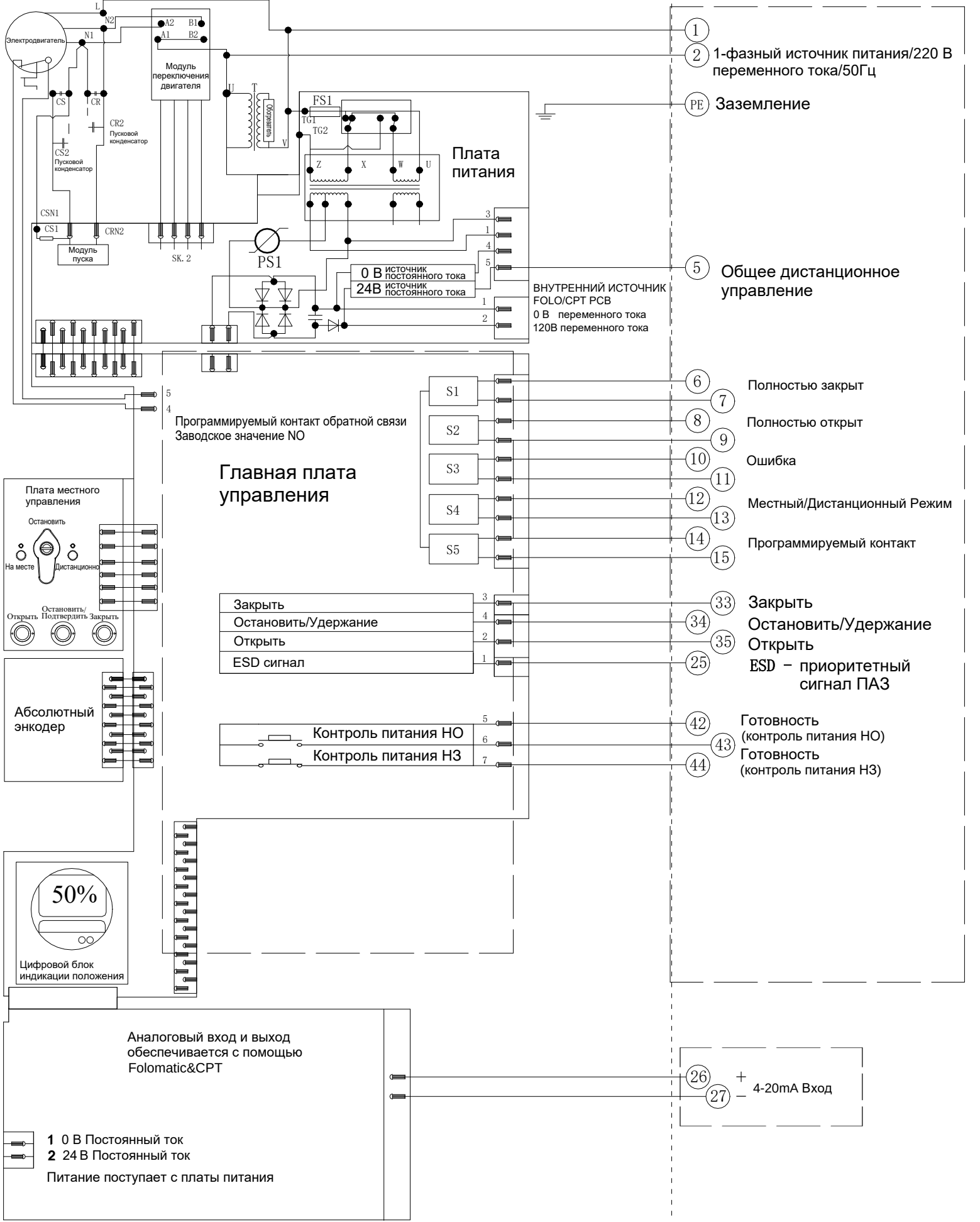
Электрическая схема №1-220-24-6-N-2 Серия VAD
