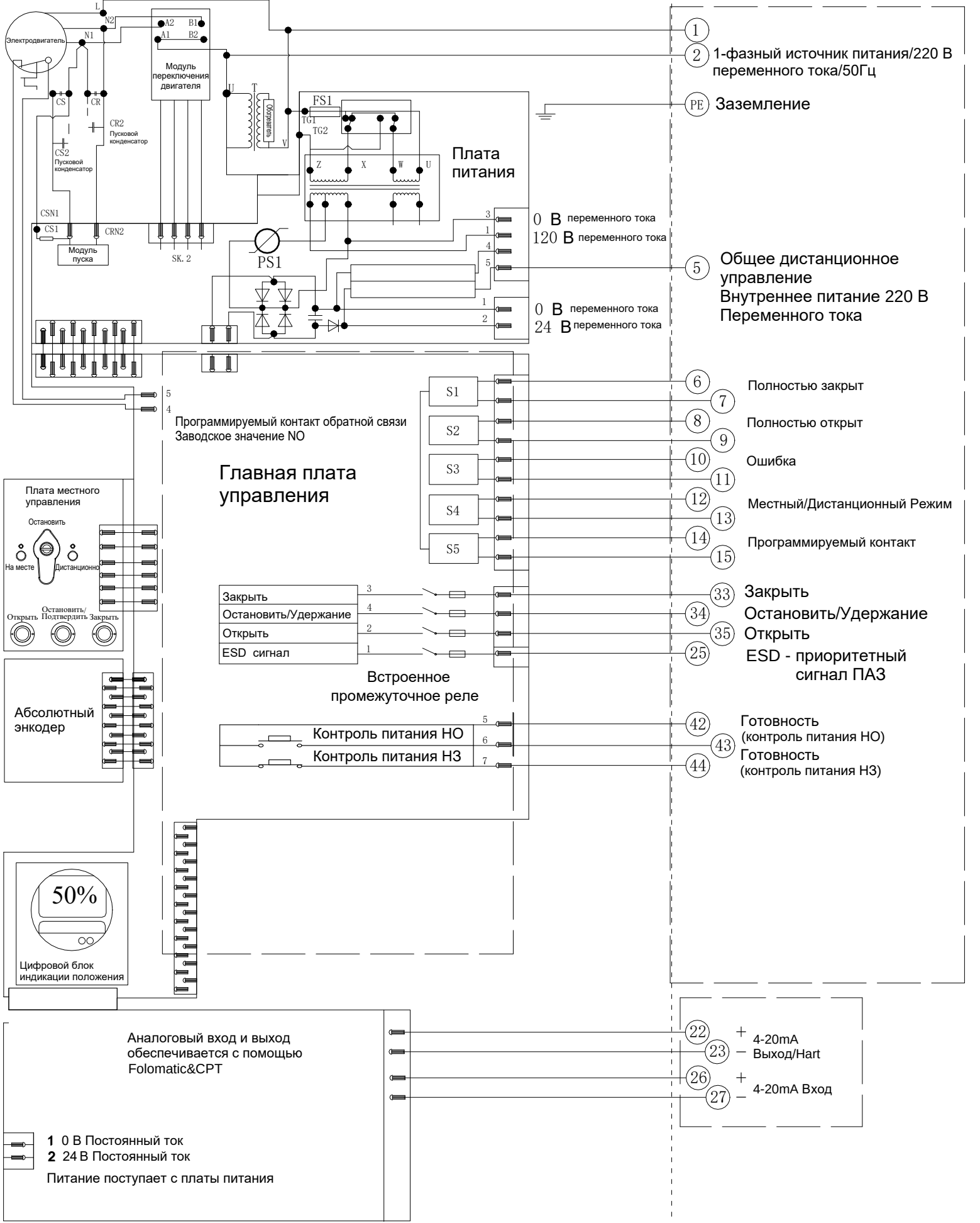
Электрическая схема №1-220-220-6-HR- 1 Серия VAD
