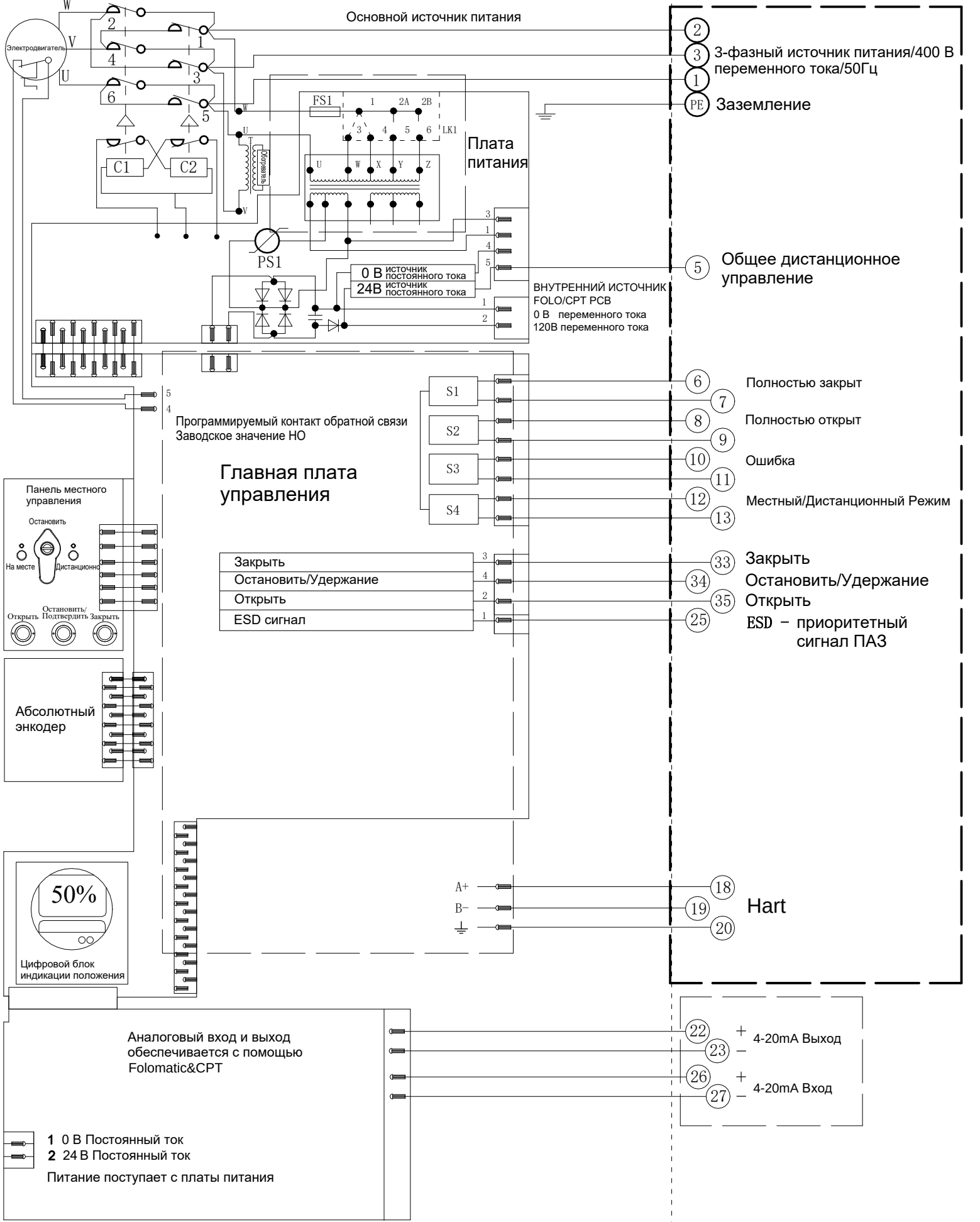
Электрическая схема №1-400-24-4-HR- 1 Серия VAD
