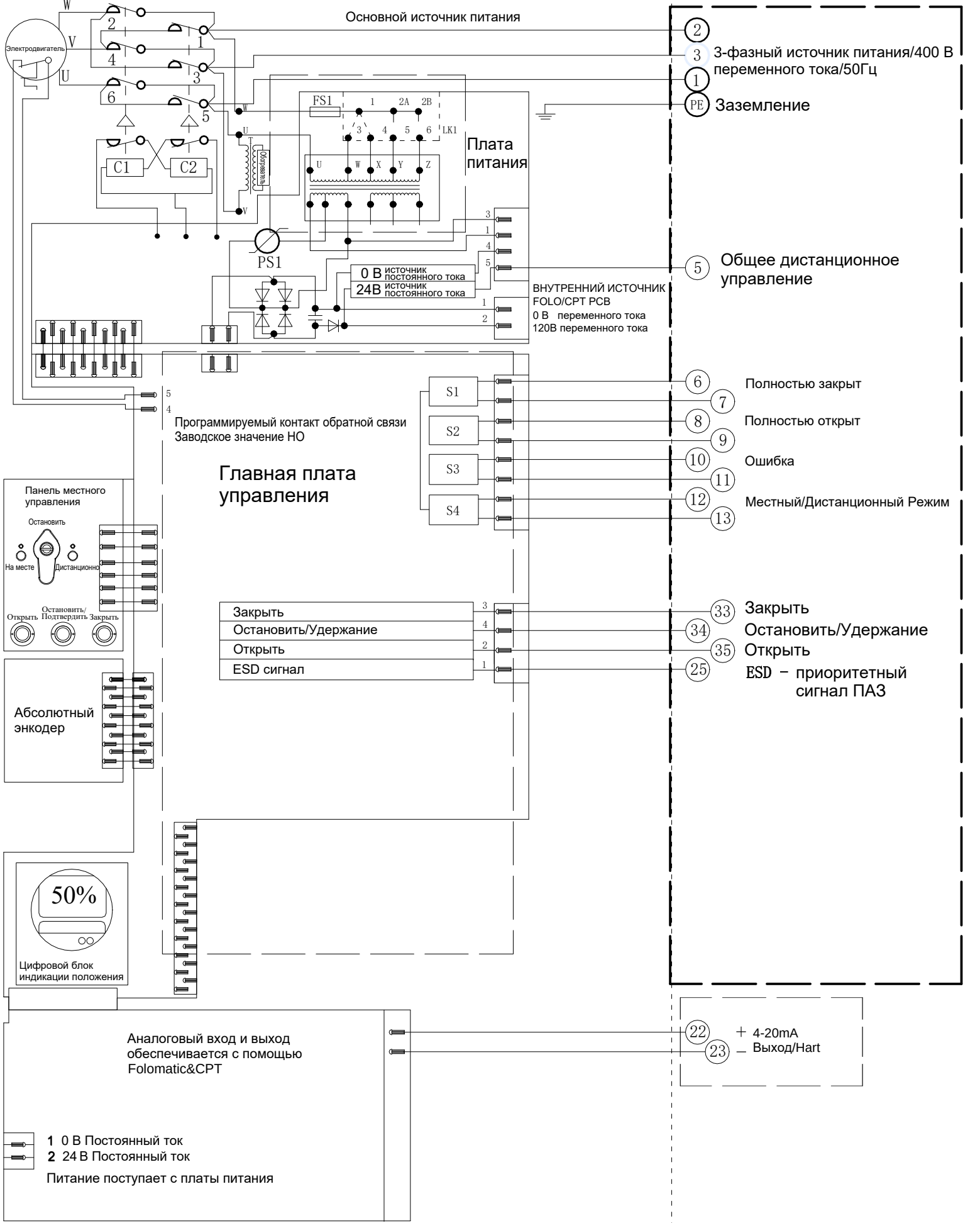
Электрическая схема №1-400-24-4-HR-3 Серия VAD
