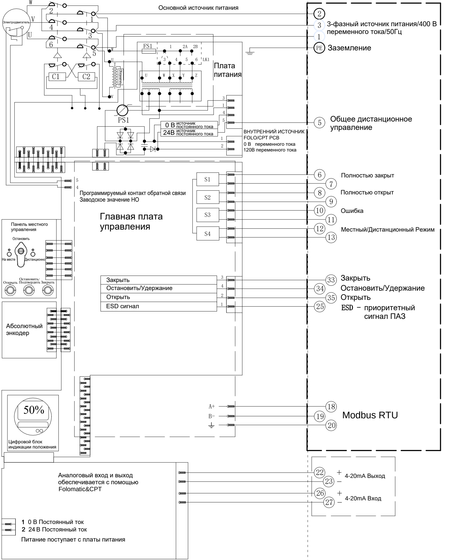
Электрическая схема №1-400-24-4-MR-1 Серия VAD
